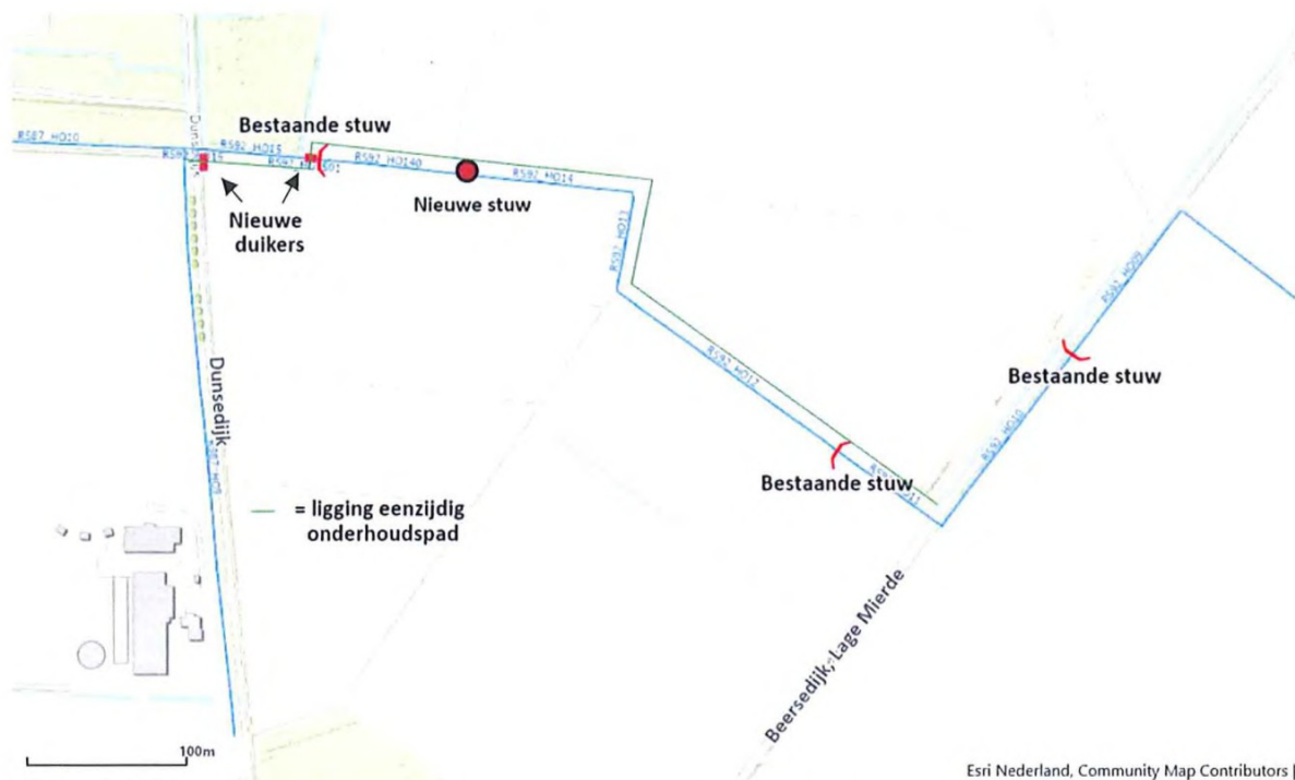
Figuur 1, Locatie nieuwe stuw (rood bolletje) in de RS92 te Lage Mierde. De twee nieuwe duikers zijn met een rode lijn aangegeven.
