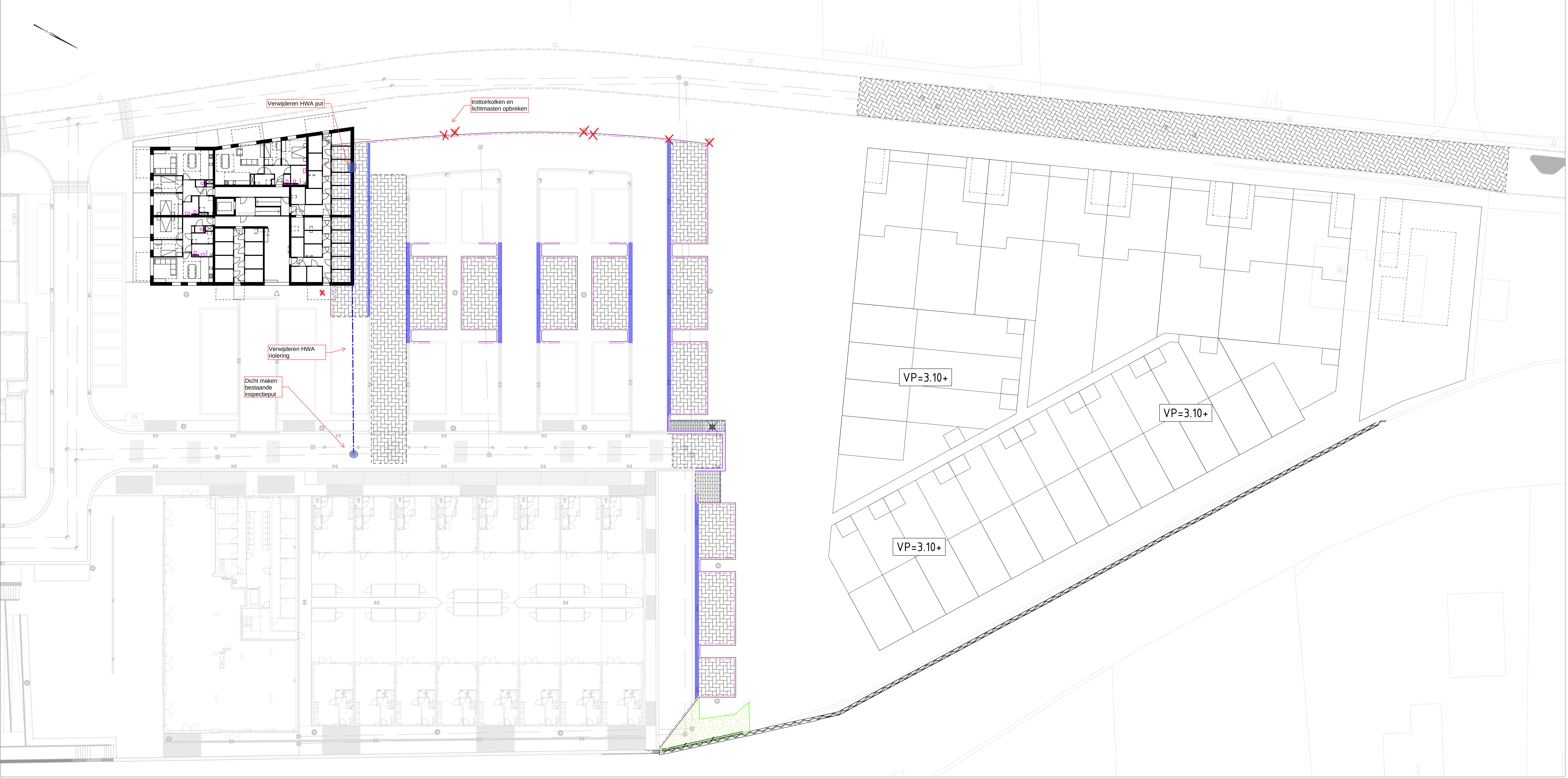
Situatieoverzicht SCHAAL 1: 200
