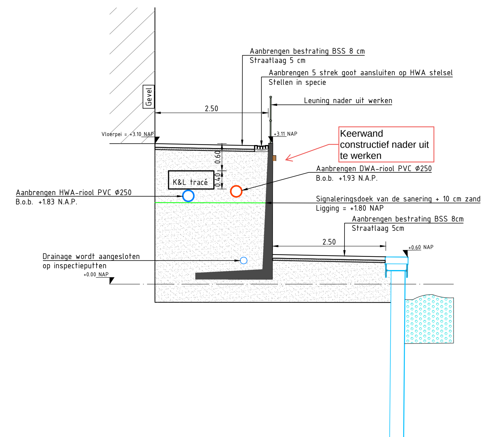
Doorsnede A-A : Voetpad / langs de Mark SCHAAL 1: 50
