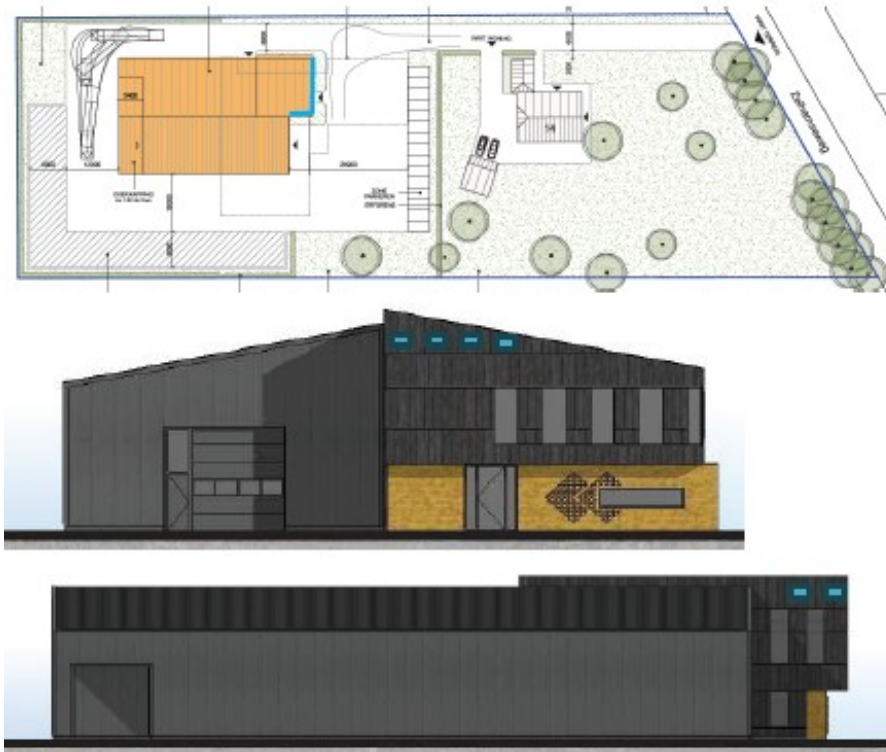
Figuur 4. Locaties van de permanente huismus verblijven op de gevel van de nieuwe loods. De huismuskasten worden geplaatst op de noord- en oostgevel.
