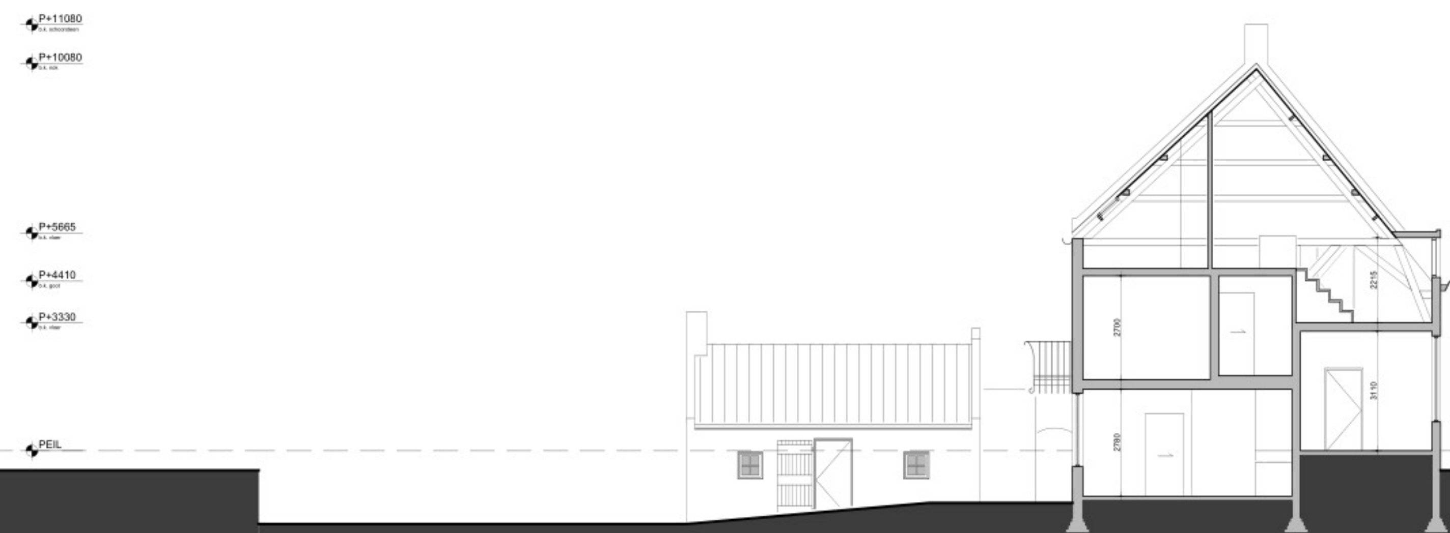
DOORSNEDE CC BESTAAND
