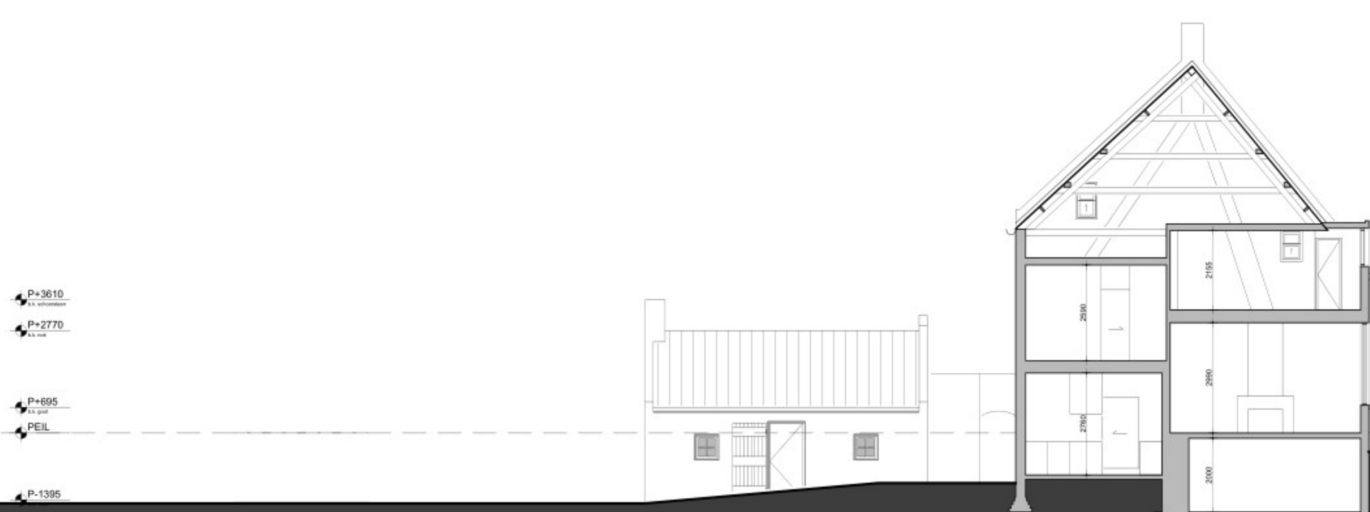
DOORSNEDE BB BESTAAND
