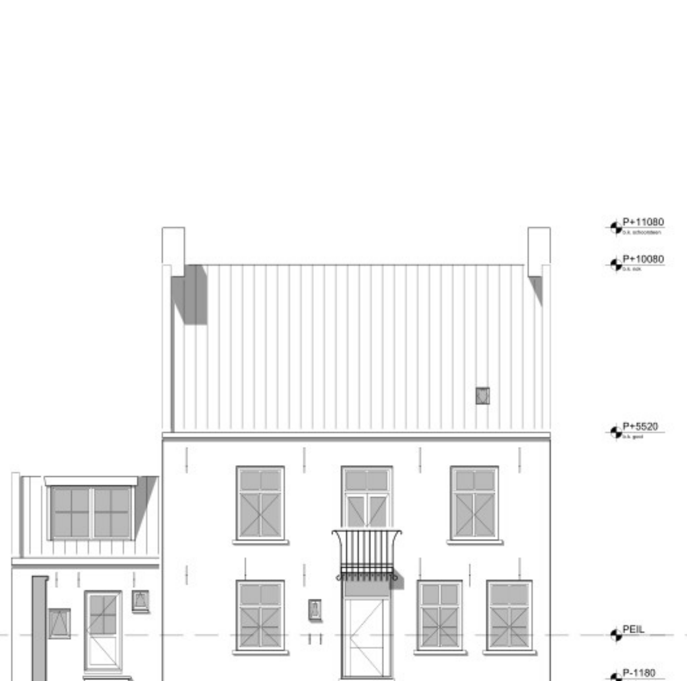
ACHTERGEVEL BESTAAND
