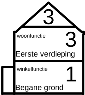
Doorsnede B schaal 1:200
