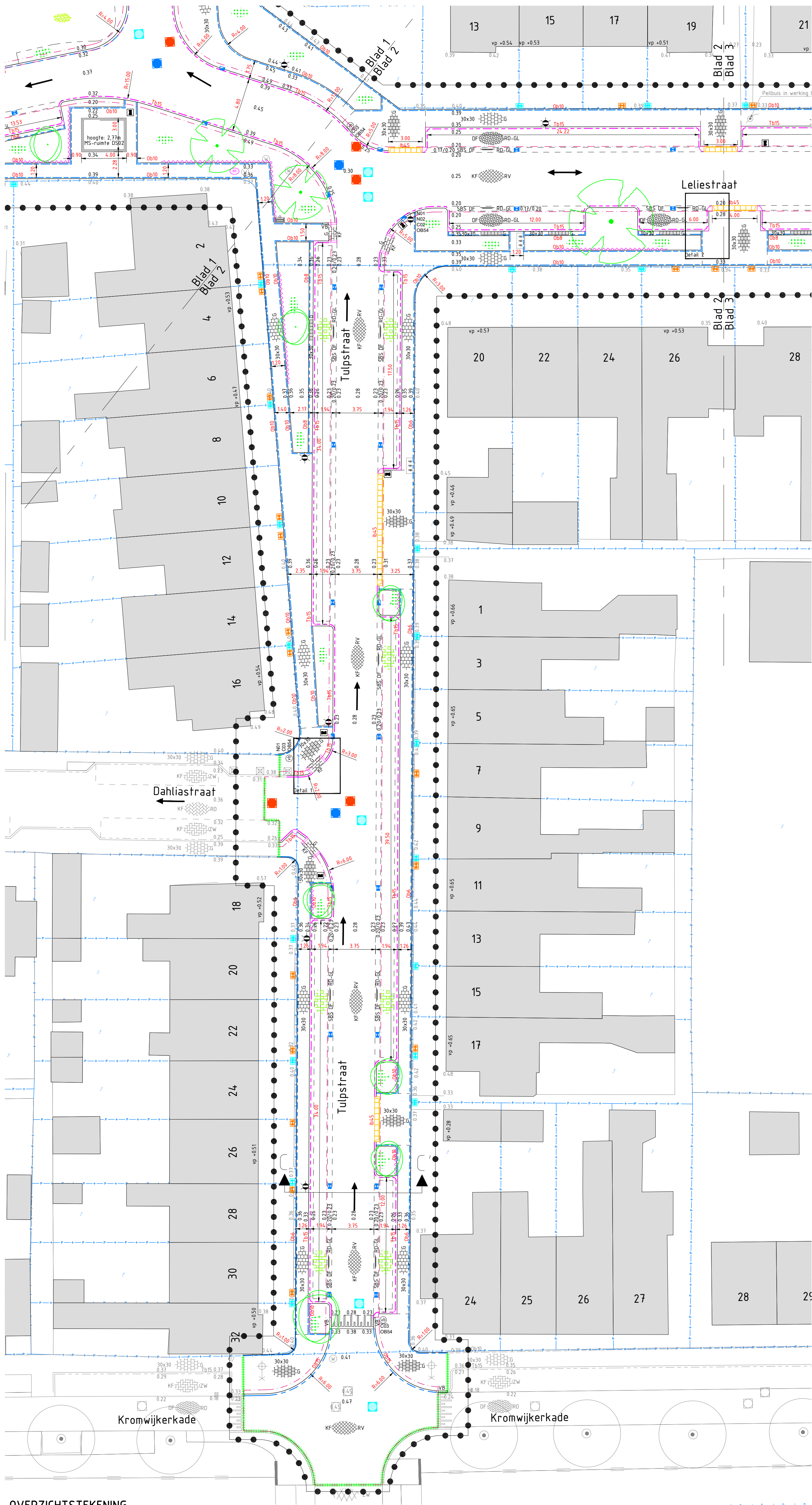
OVERZICHTSTEKENING SCHAAL 1:200
