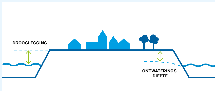
Figuur 5: Verschil tussen drooglegging (maaiveld t.o.v. waterpeil) en ontwateringsdiepte (maaiveld t.o.v. grondwaterstand).
