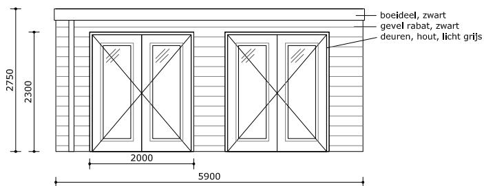
Gevelaanzicht Fagelstraat
