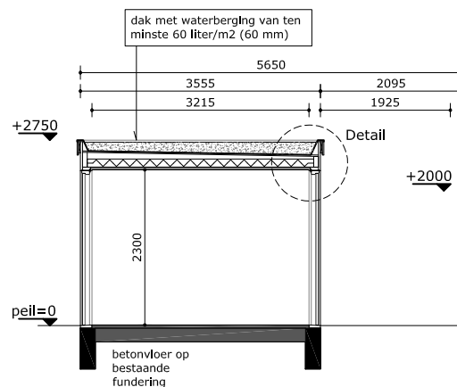
Doorsnede
