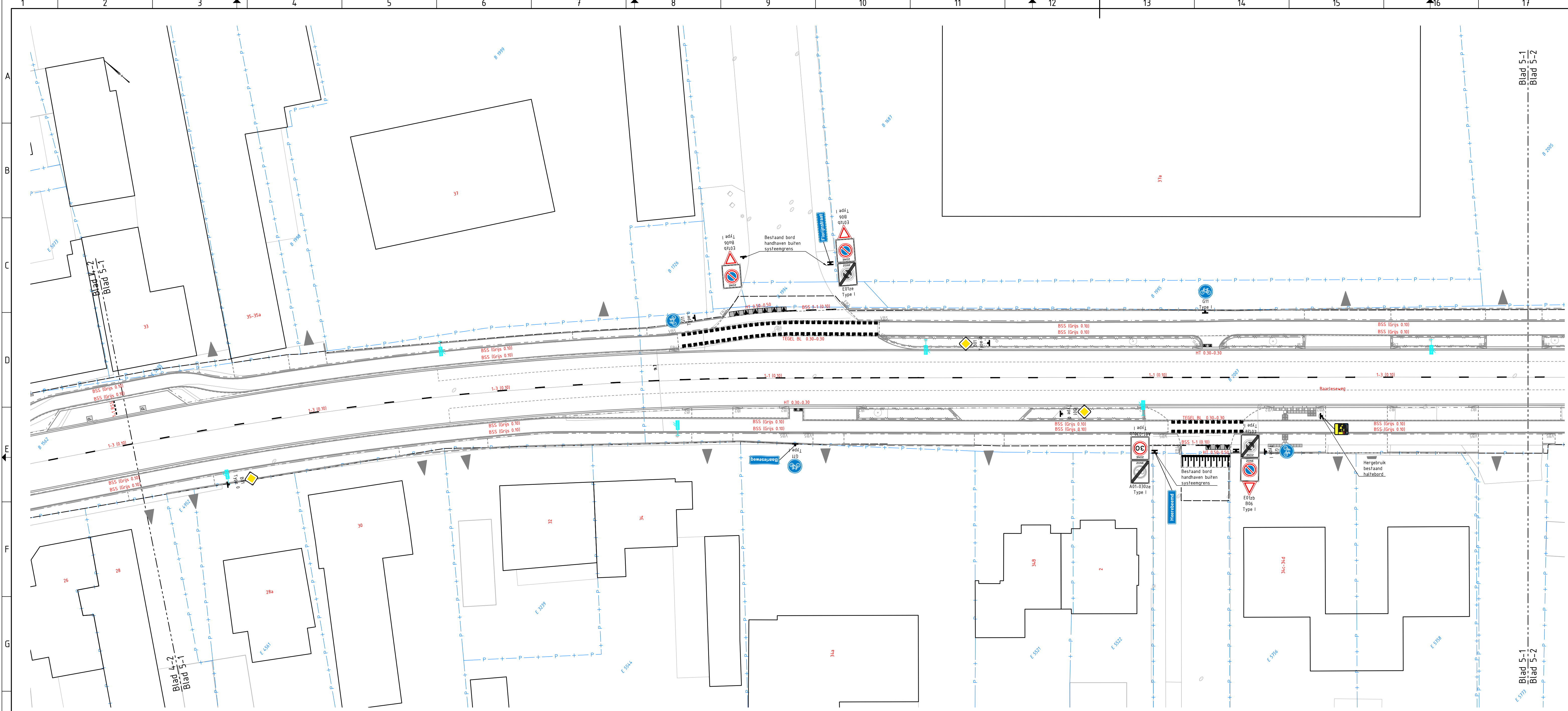
SITUATIE: BLAD 5-1 SCHAAL 1 : 200
