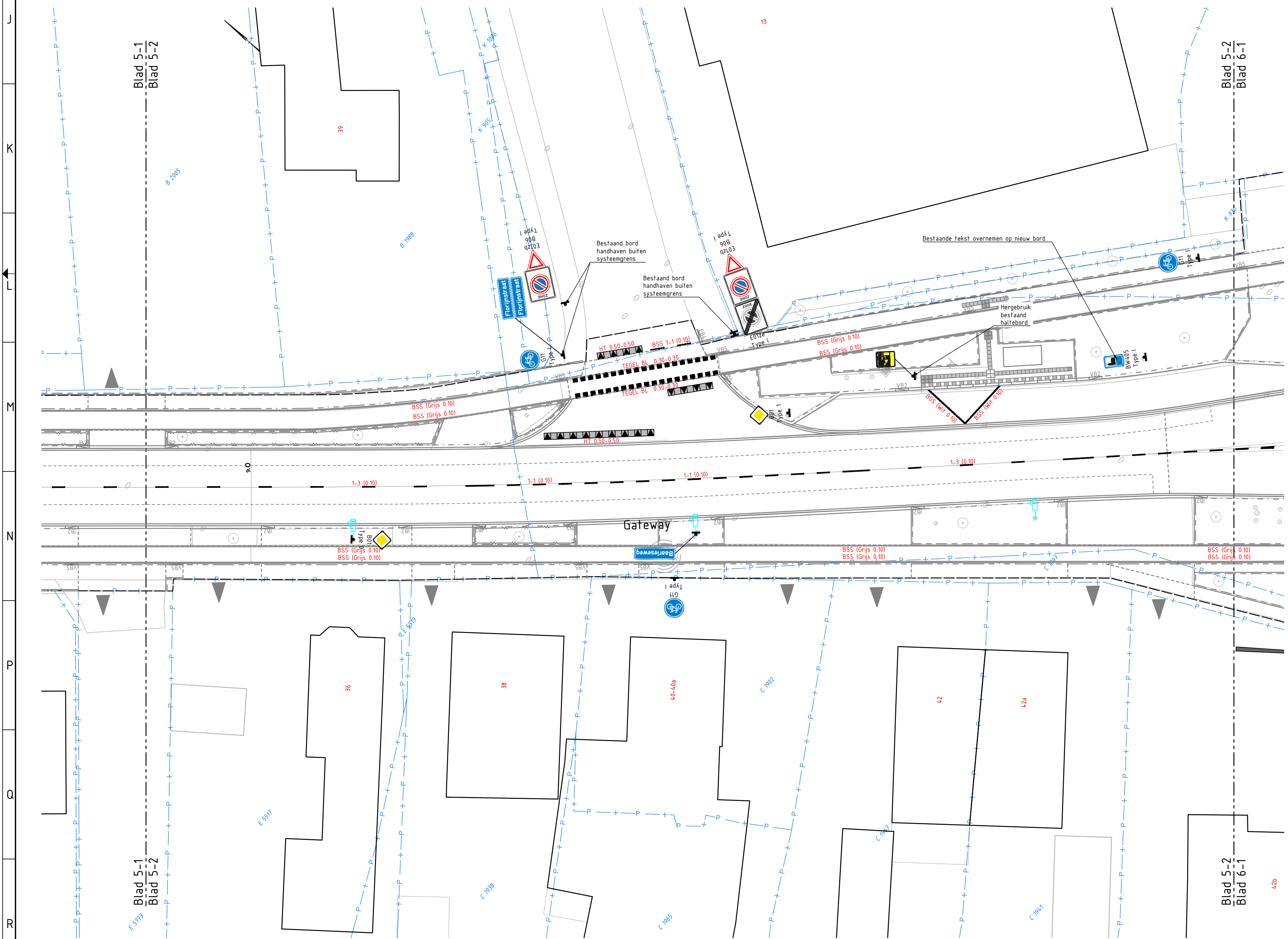
SITUATIE: BLAD 5-2 SCHAAL 1 : 200
