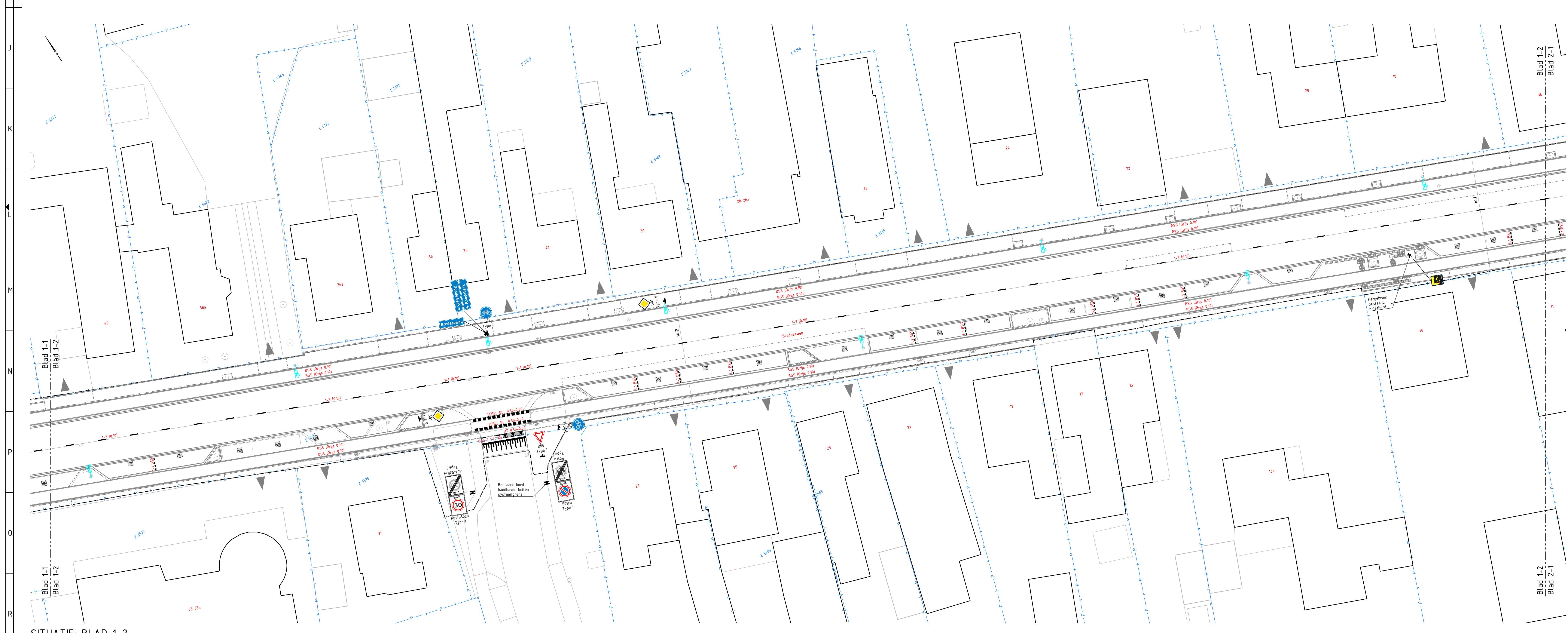
SITUATIE: BLAD 1-2 SCHAAL 1: 200
