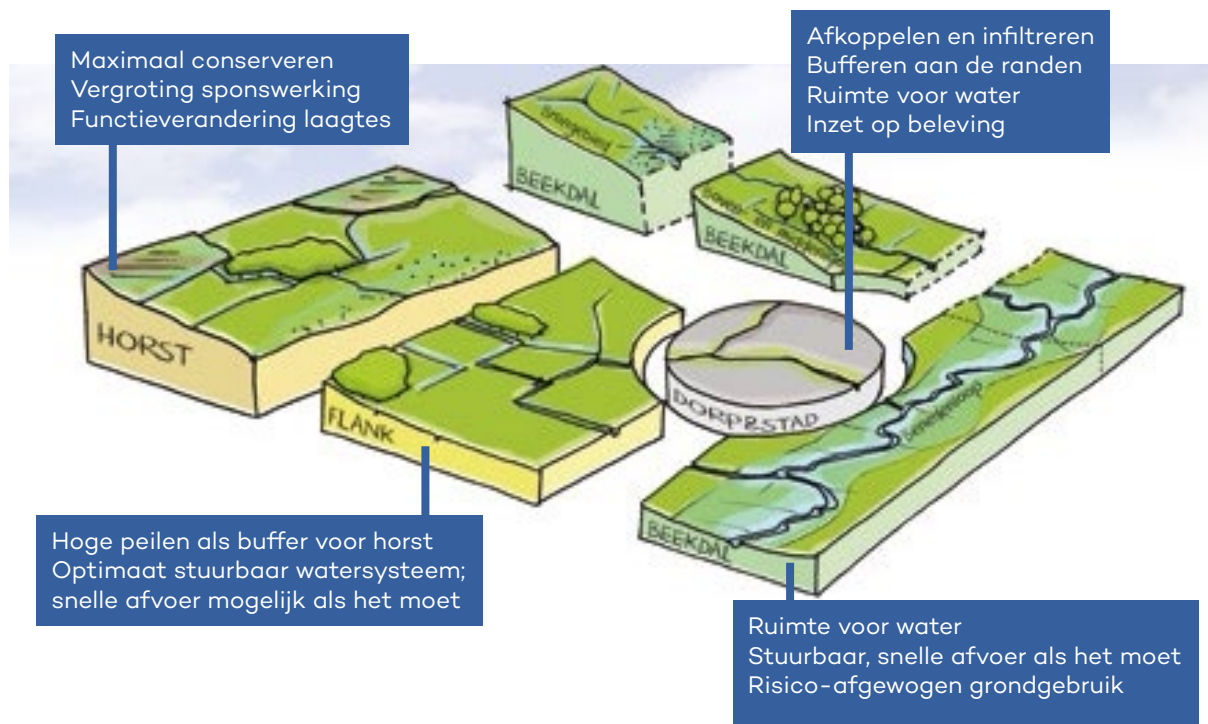
Afbeelding 15. Het verhaal van de Aa: principes en bouwstenen voor een klimaatrobuust watersysteem.
