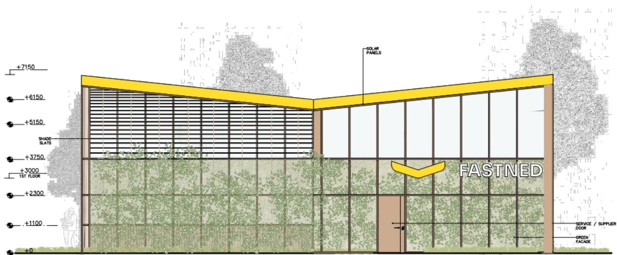
BACK ELEVATION 1:150
