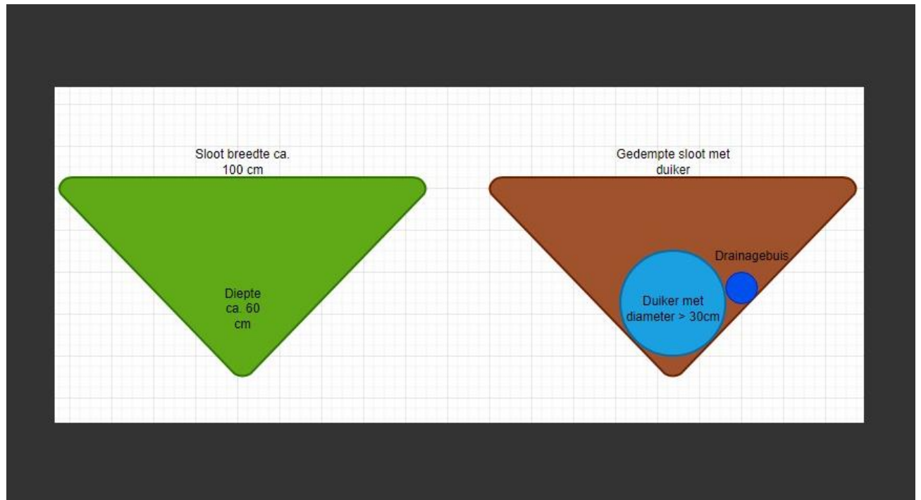
Tekening 855220-C
