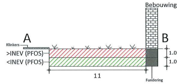
Dwarsdoorsnede Schaal 1:250
