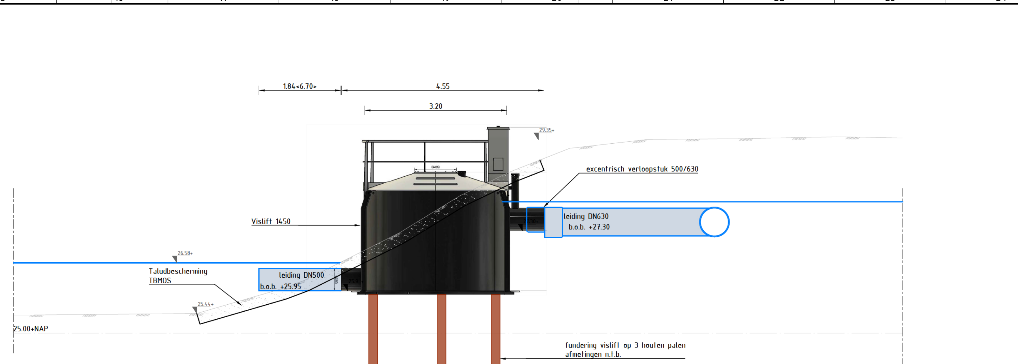
Dwarsprofiel A schaal 1:50
