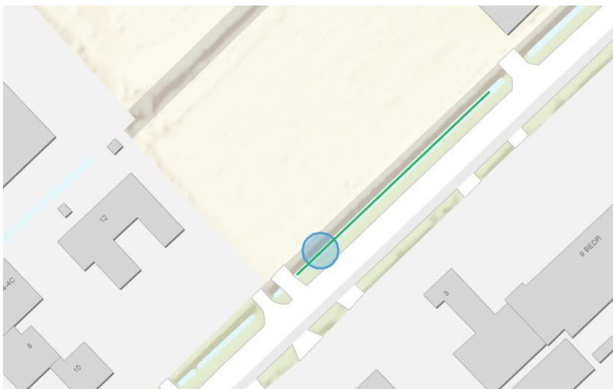
Figuur 1: De blauwe cirkel geeft de locatie van de aan te leggen dam met duiker weer. De groene lijn geeft de locatie weer van de watergang die verbreed dient te worden.
