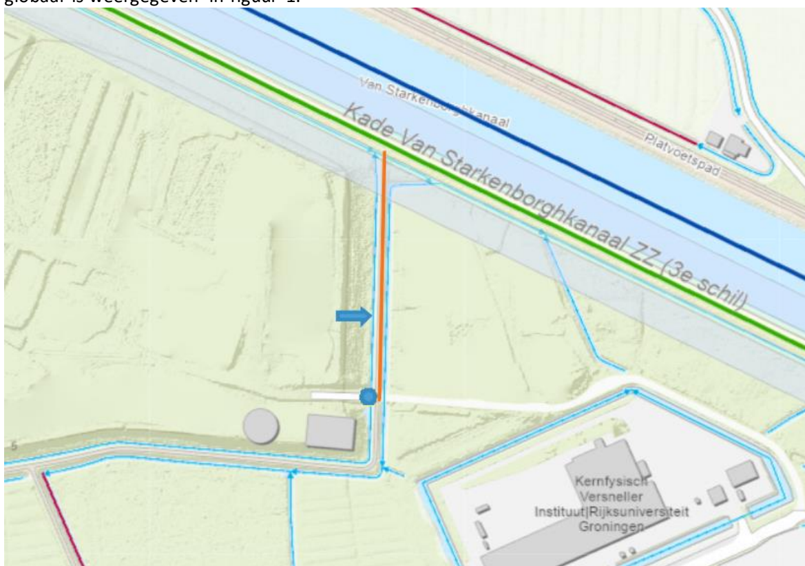
Figuur 1: Het te verbreden fietspad is weergegeven met de oranje lijn, de te leggen duiker in de toegangsdam is weergegeven met de blauwe cirkel en de aan te passen watergang is weergegeven met de blauwe pijl.
