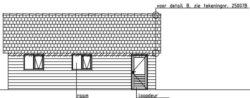
RECHTERGEVEL
