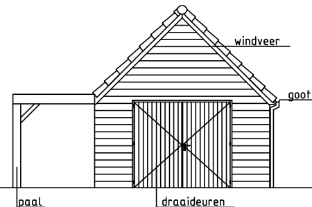
VOORGEVEL
