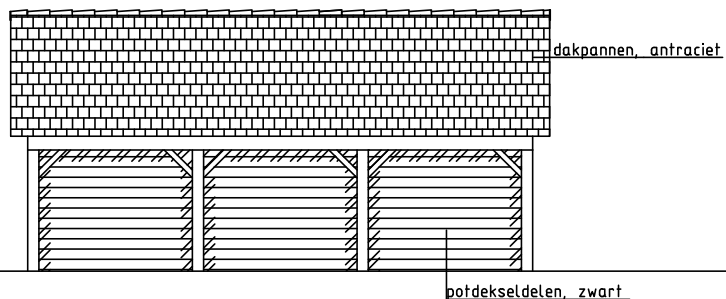
LINKERGEVEL
