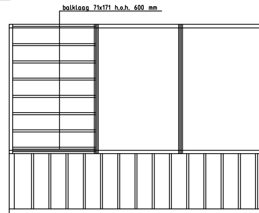
VERDIEPINGSVLOER
