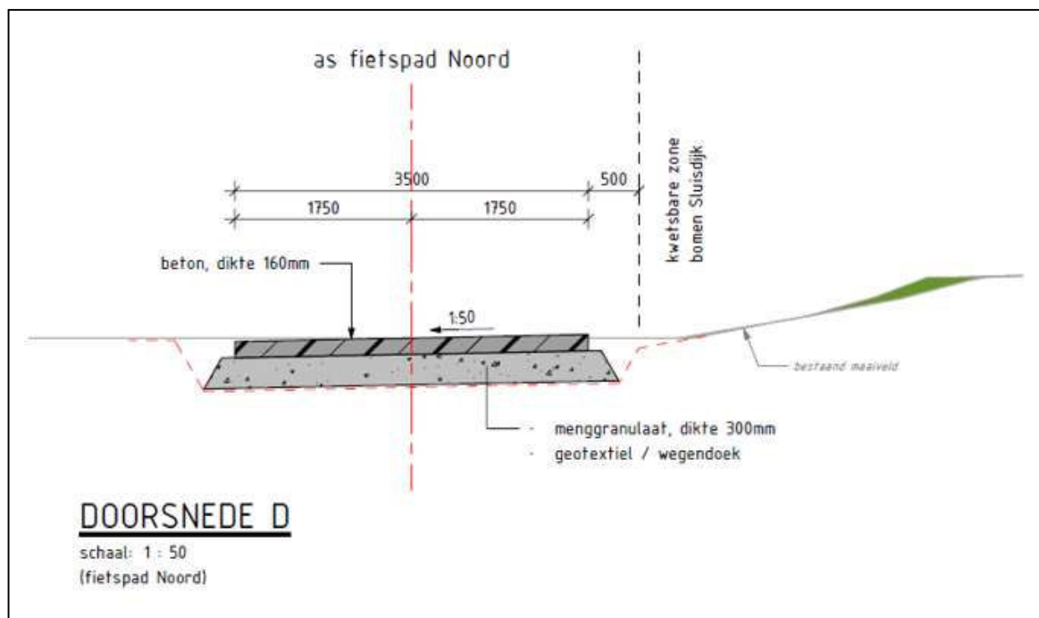
Figuur 2: Dwarsprofiel fietspad op de noordelijke oever
