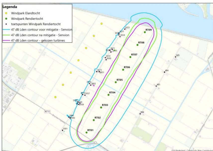
Afbeelding 3.1 47 dB Lden geluidscontour van windpark Rendiertoht berekend met de Senvion turbine (voor en na mitigatie) en de uiteindelijk gekozen turbines (Vestas V162-5.6 én V162-6.0 MW)
