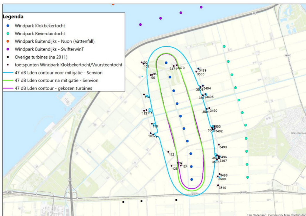
Afbeelding 3.1 47 dB Lden geluidscontour van windpark Klokbeektocht/Vuursteentocht berekend met de Senvion turbine (voor en na mitigatie) en de uiteindelijk gekozen turbines (Vestas V162-5.6 én V162-6.0 MW)
