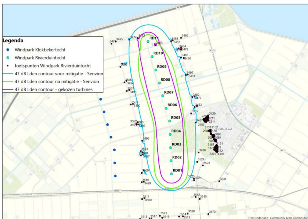
Afbeelding 3.1 47 dB Lden geluidscontour van windpark Rivierduintoicht berekend met de Senvion turbine (voor en na mitigatie) en de uiteindelijk gekozen turbines (Vestas V162-5.6 én V162-6.0 MW)
