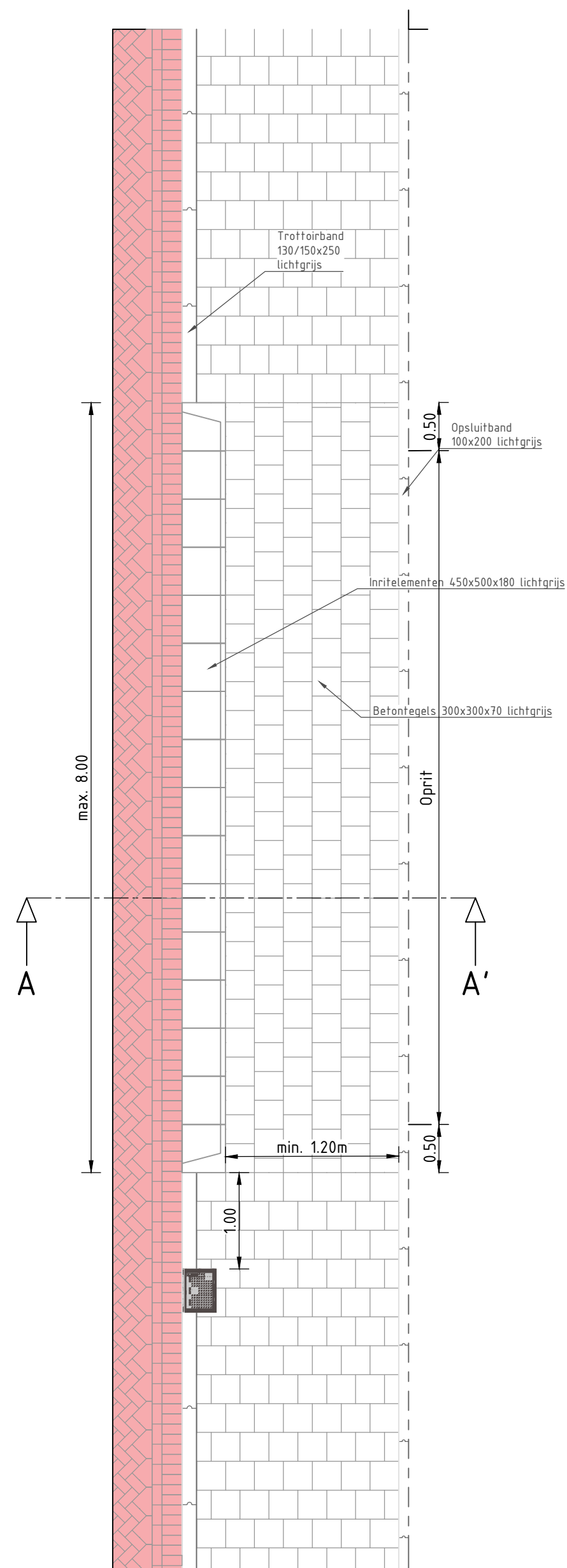
Principe detail uitrit maatschappelijke voorziening / bedrijf Wel vrachtverkeer op eigen terrein
