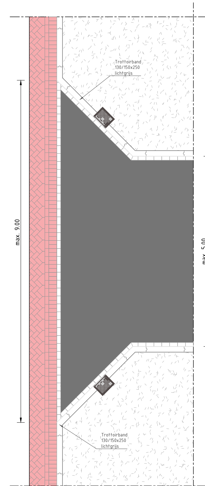
Principe detail uitrit landbouwperceel
