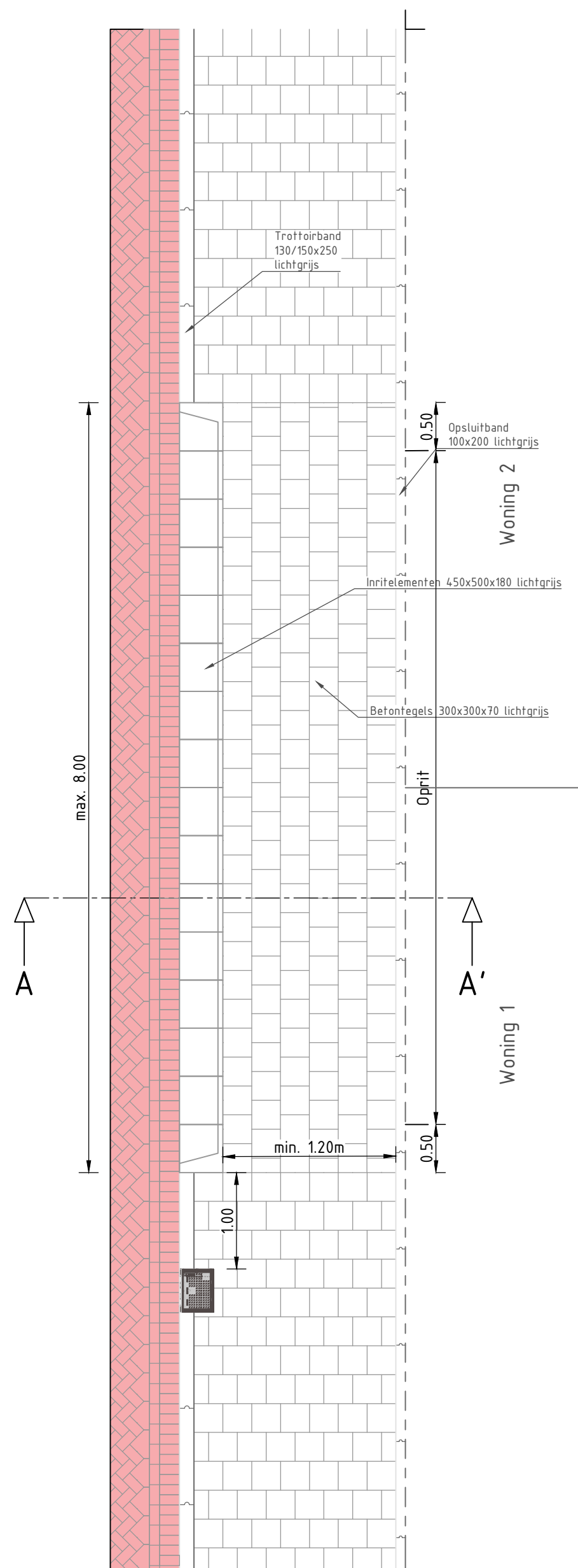
Principe detail gecombineerder particuliere inrit
