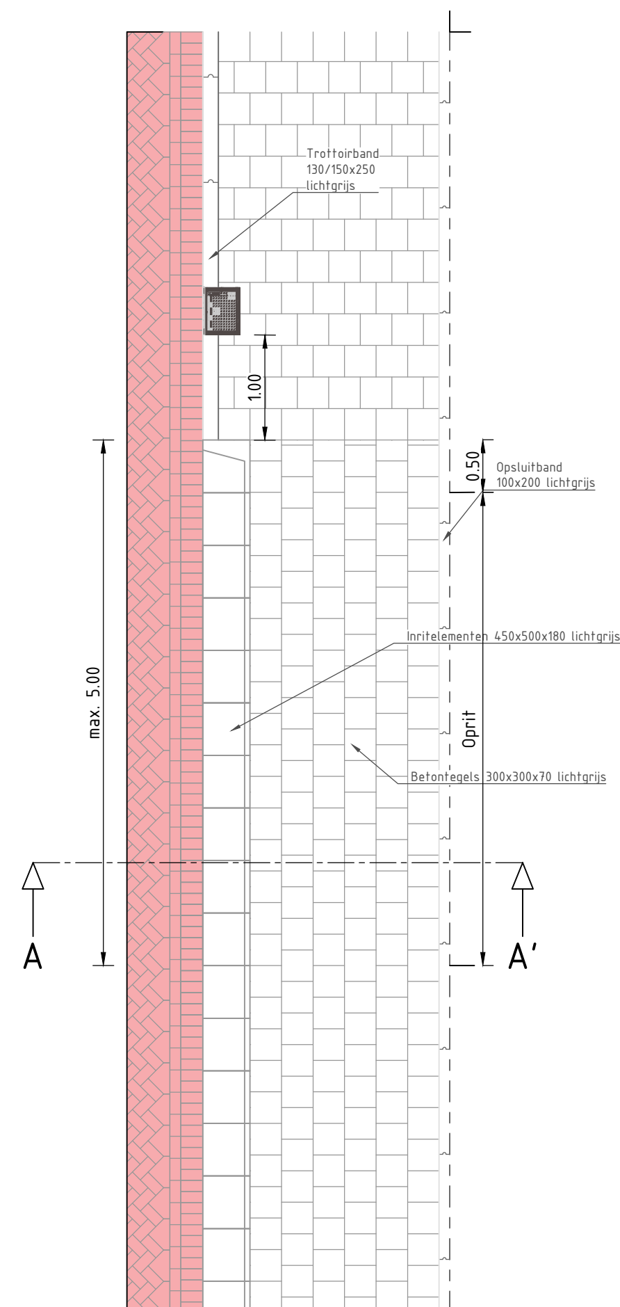
Principe detail uitrit maatschappelijke voorziening / bedrijf Geen vrachtverkeer op eigen terrein
