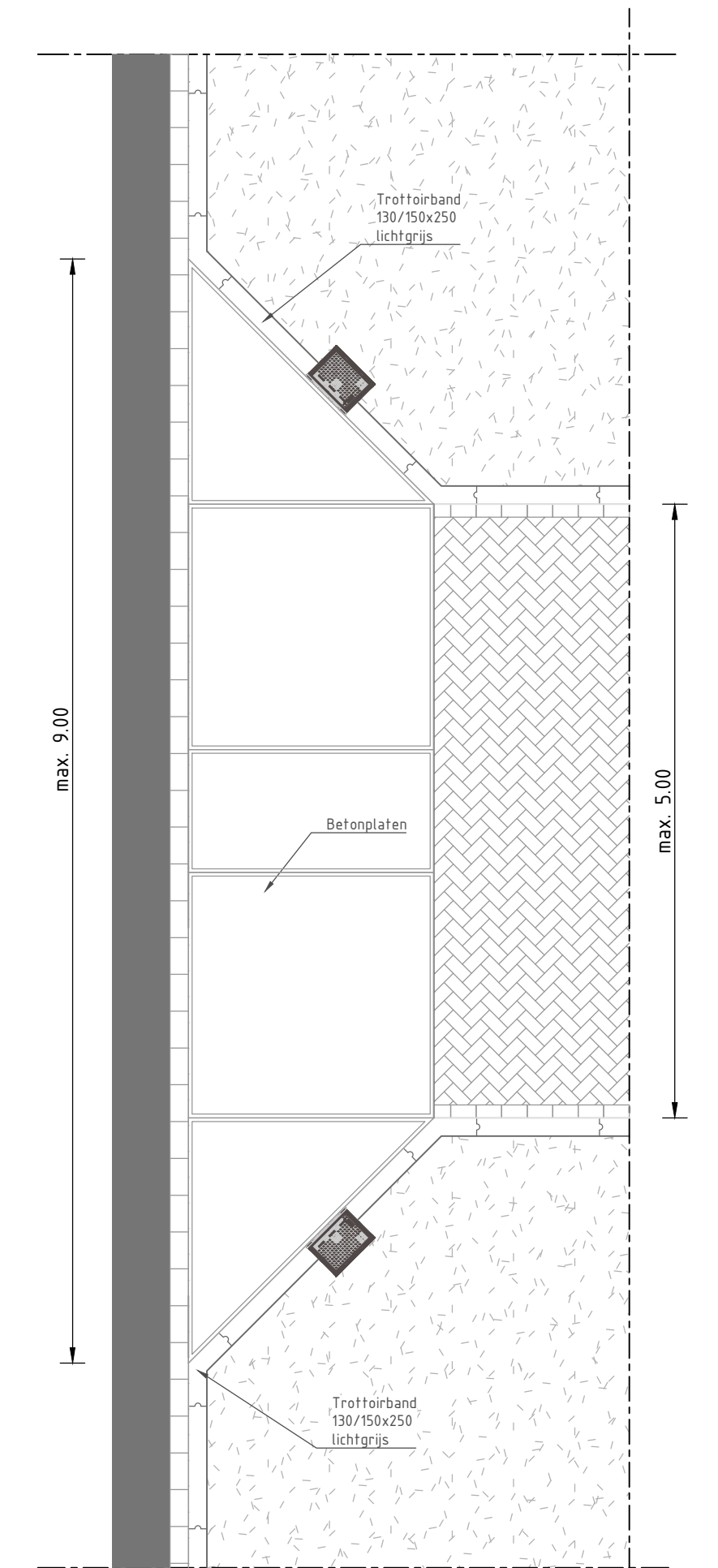
Principe detail uitrit landbouwperceel
