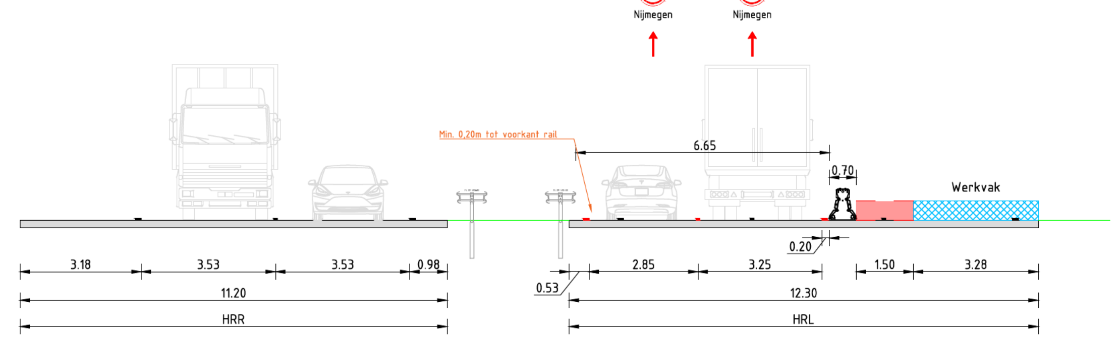
DOORSNEDE D SCHAAL 1:100 km03.3
