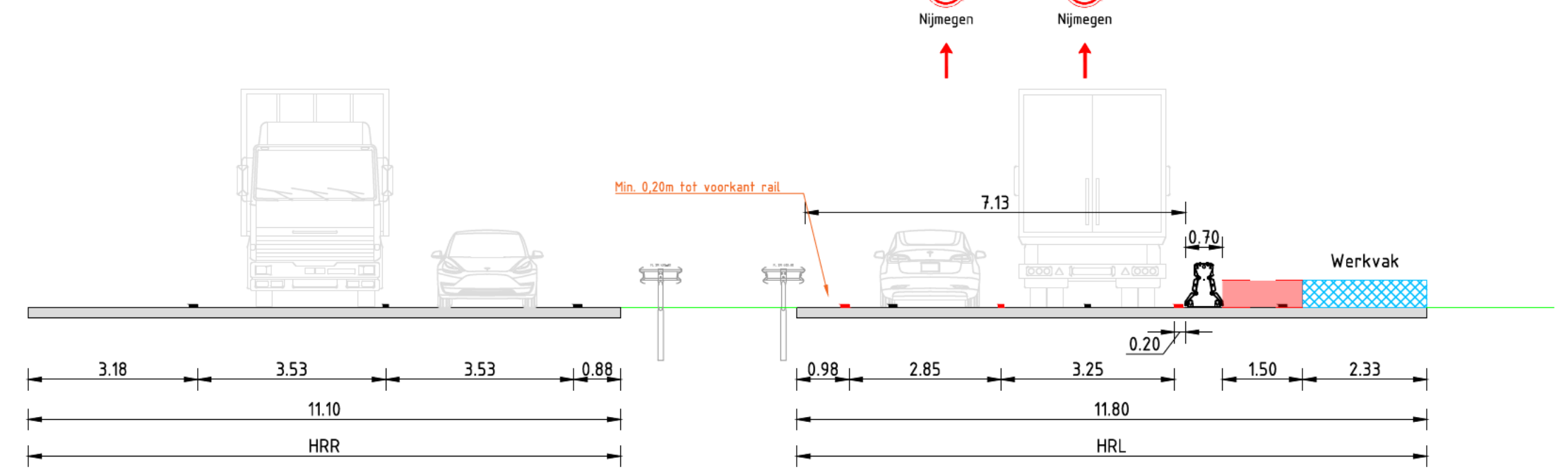
DOORSNEDE E SCHAAL 1:100 km02.96
