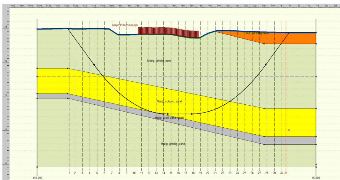
Figuur 2 Schematische weergave bodemopbouw
