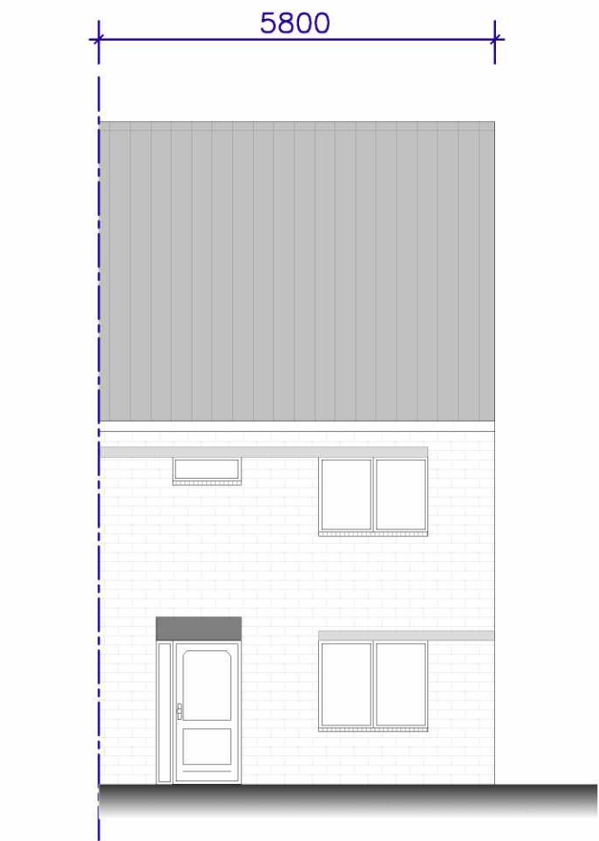
VOORGEVEL BESTAAND
