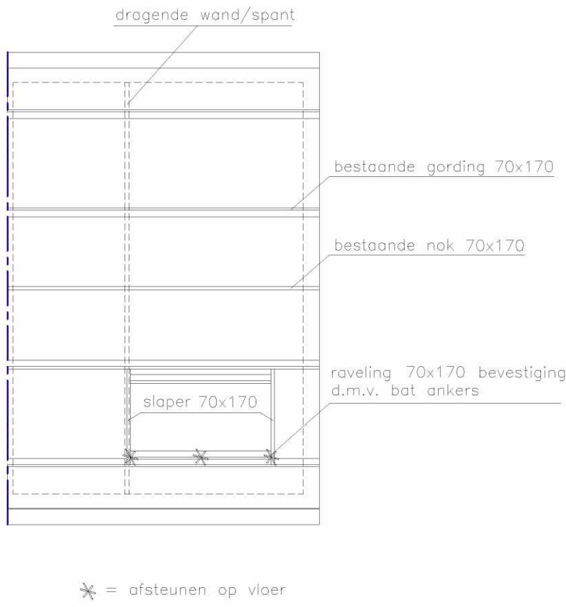
KAPPLAN NIEUW
