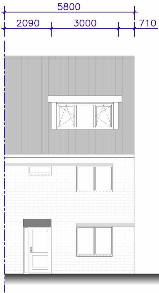
VOORGEVEL NIEUW
