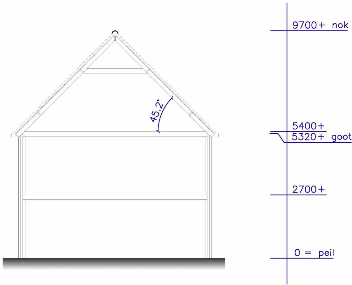
DOORSNEDE BESTAAND
