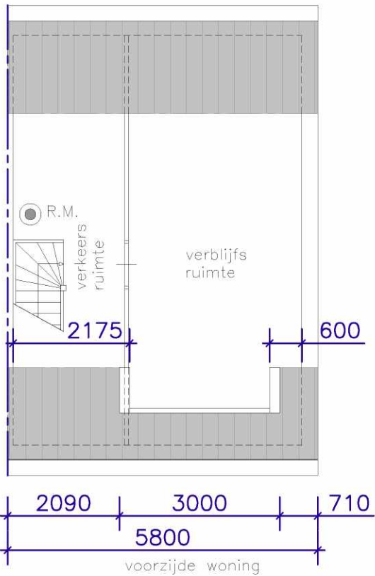
INDELING NIEUW
