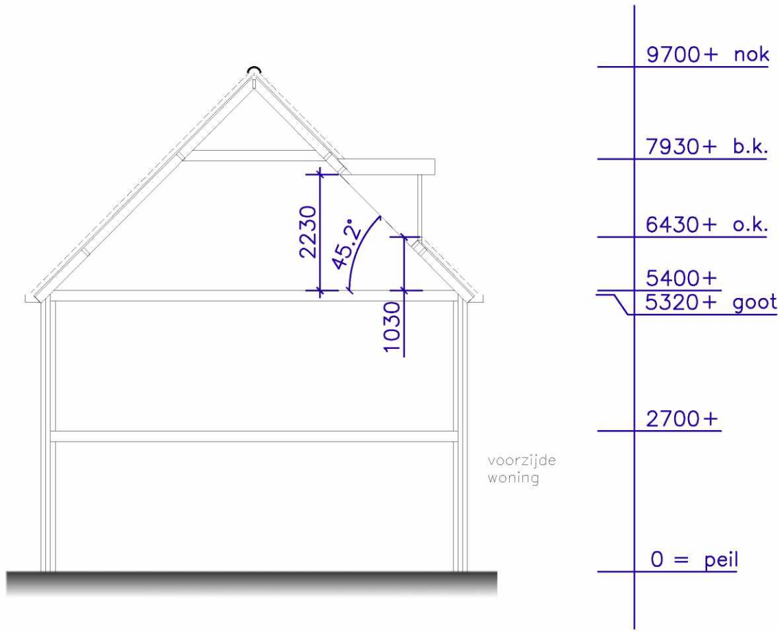
DOORSNEDE NIEUW
