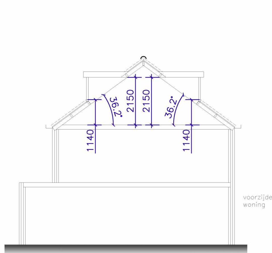
DOORSNEDE NIEUW
