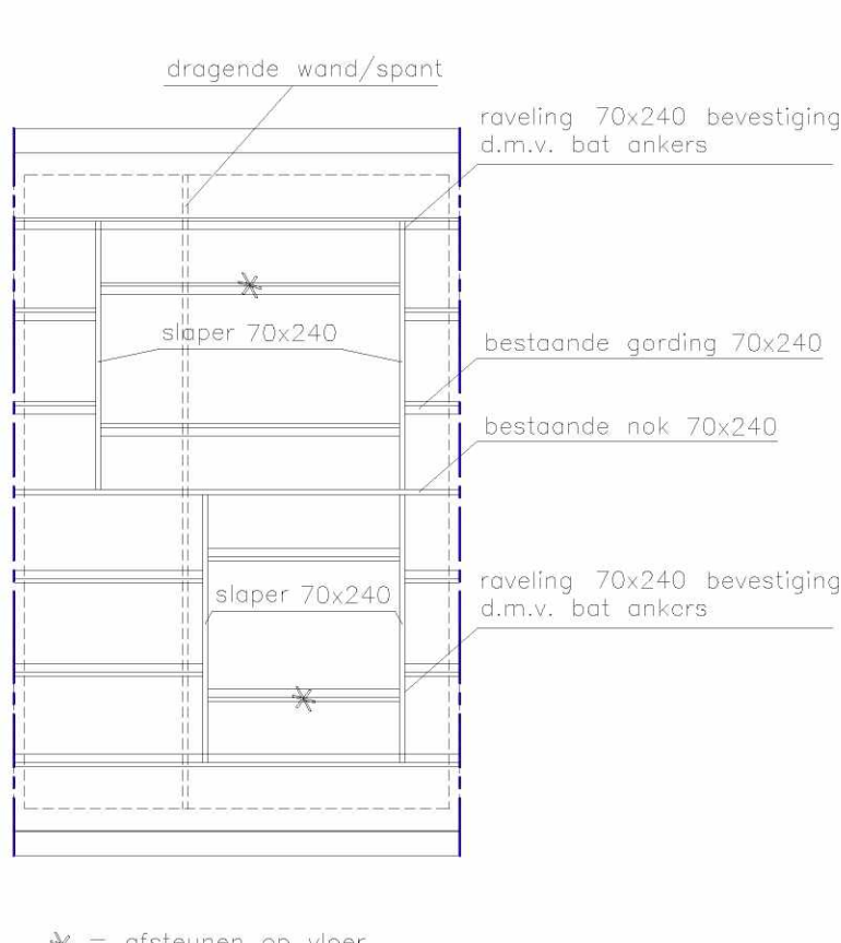
KAPPLAN NIEUW
