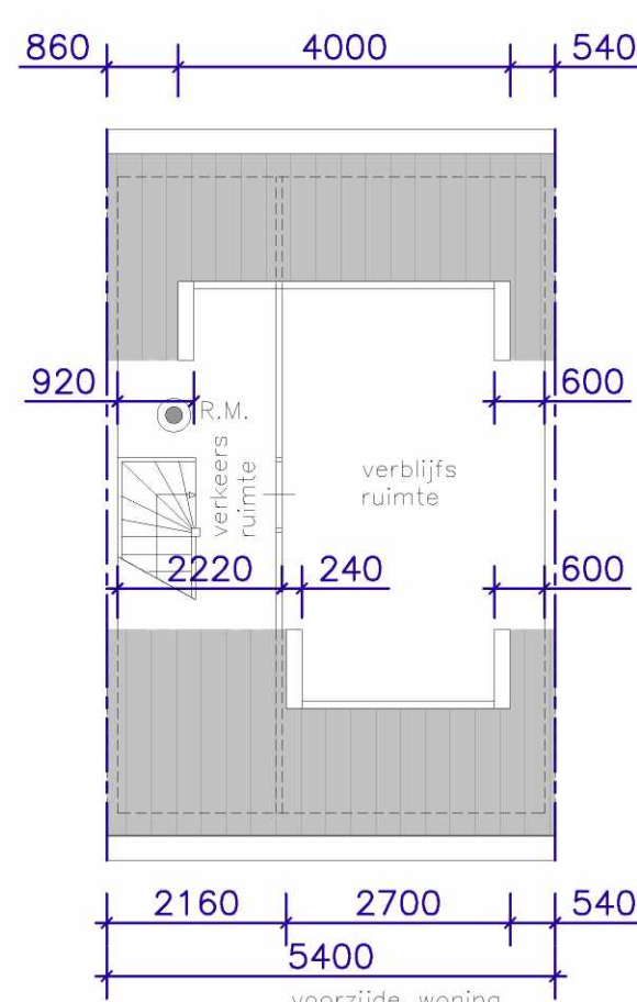
INDELING NIEUW
