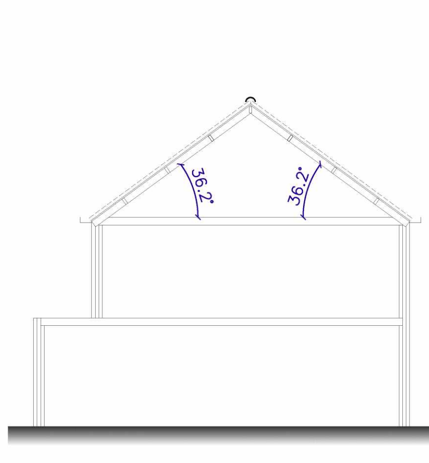
DOORSNEDE BESTAAND
