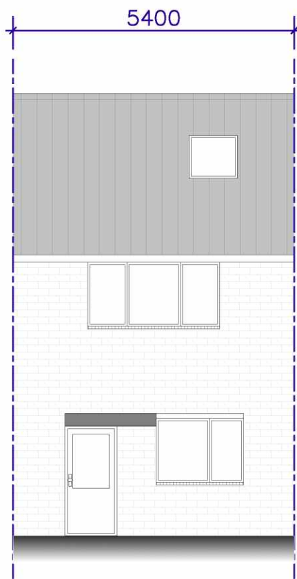
VOORGEVEL BESTAAND
