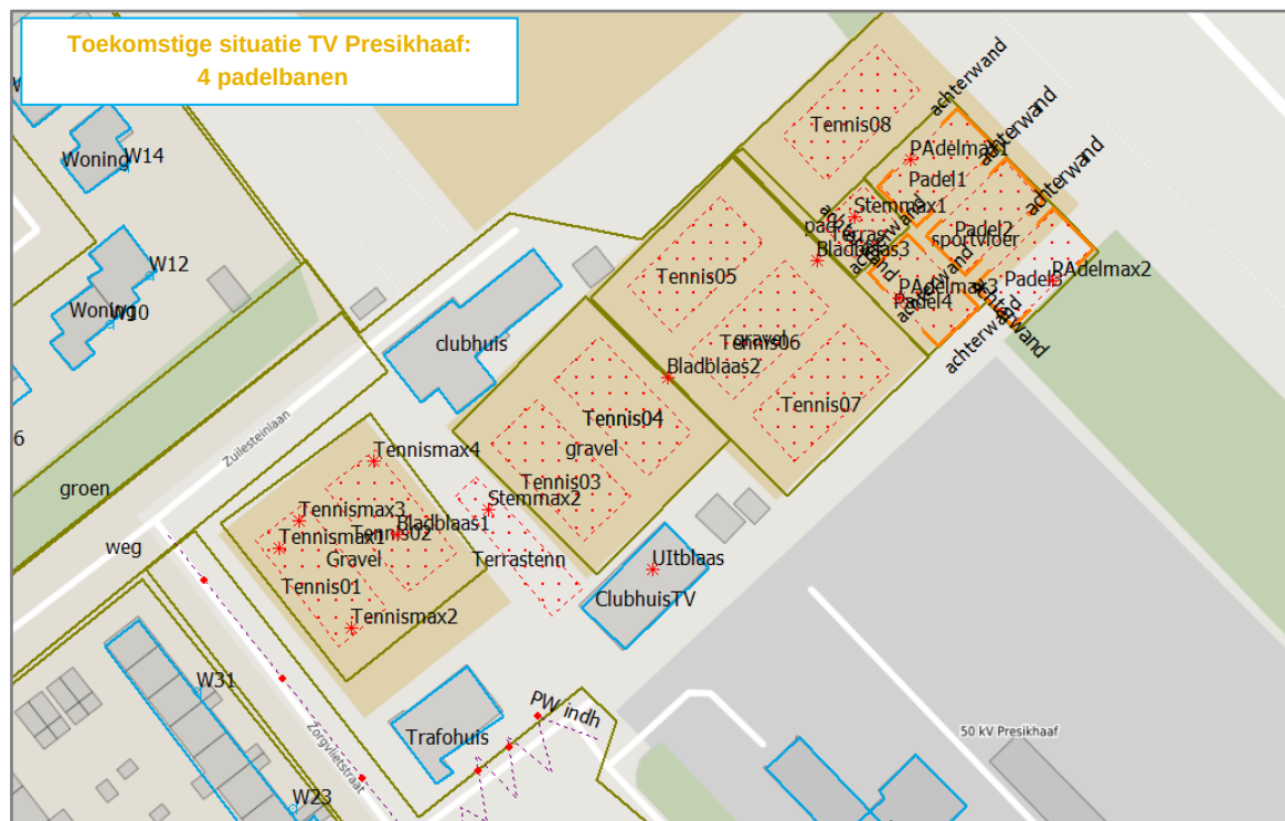
Figuren 2.3 Rekenmodel TV Presikhaaf 8x tennis en 4x padel
