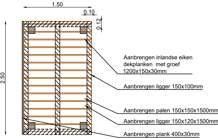
Bovenaanzicht aanlegsteiger trekpont Schaal: 1:50
