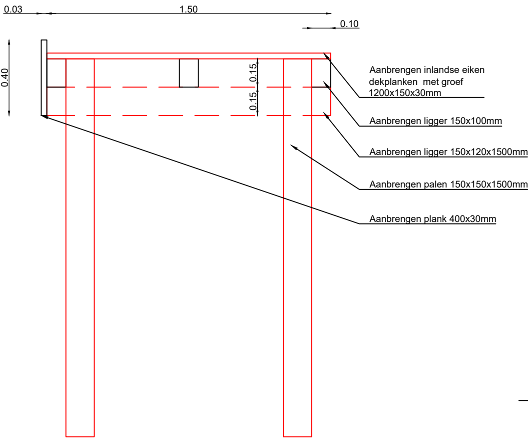
Doorsnede aanlegsteiger trekpont Schaal: 1:20
