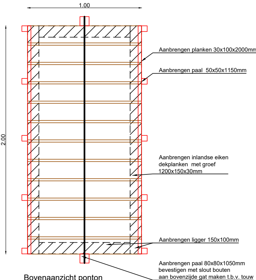
Bovenaanzicht ponton Schaal: 1:20
