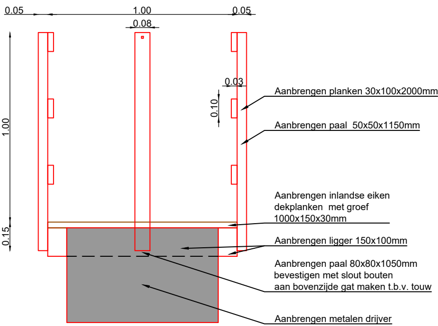
Doorsnede ponton Schaal: 1:20
