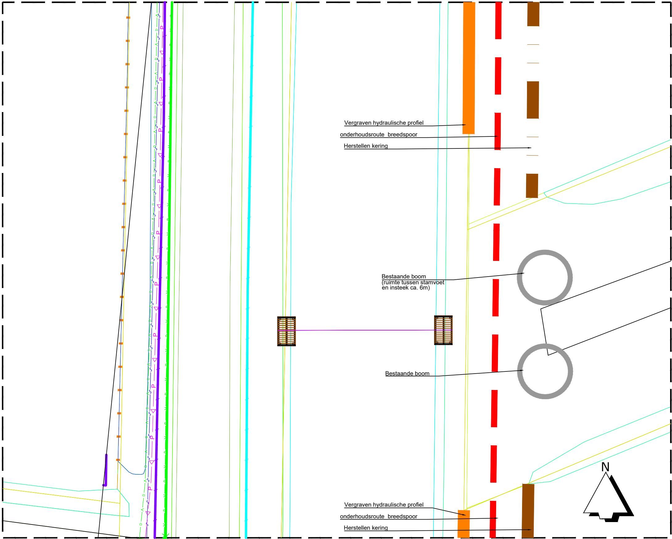
Detail Trekpont Schaal: 1:200
