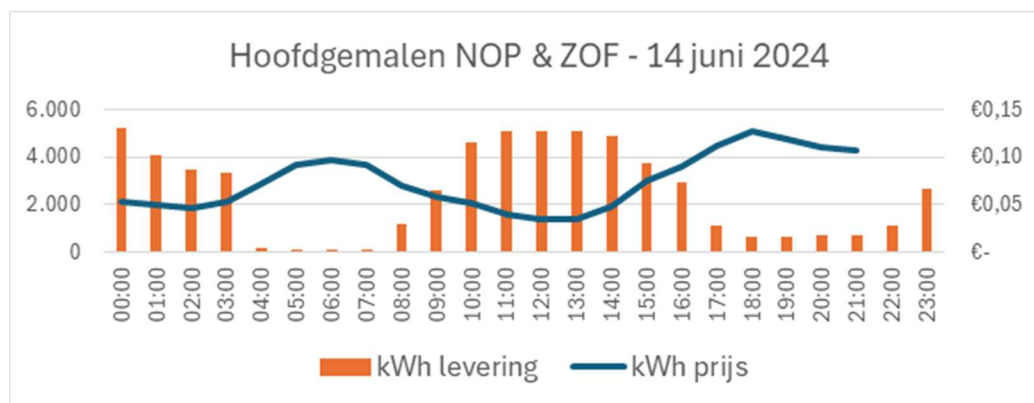
Figuur 18 Ter illustratie: energie bemaling versus energieprijzen op 14 juni 2024, waaruit blijkt dat we malen op momenten dat de prijs laag is.
