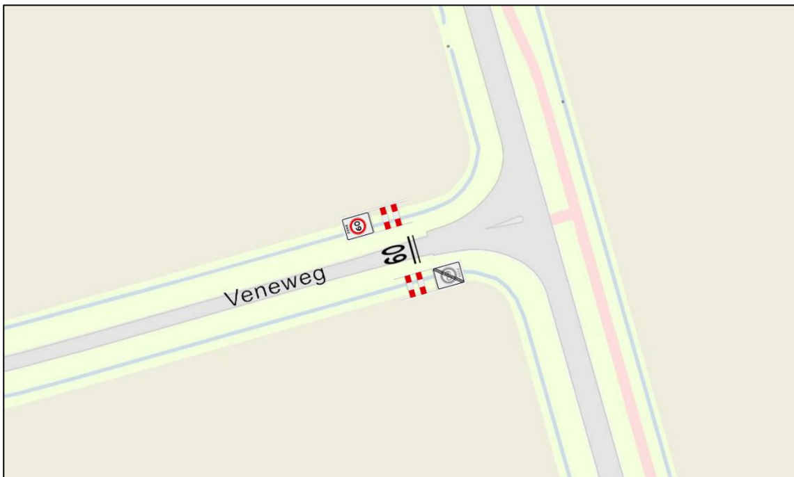
Detail 2 (Aanbrengen portalen, dwarsmarkeringen en 60-markering)
