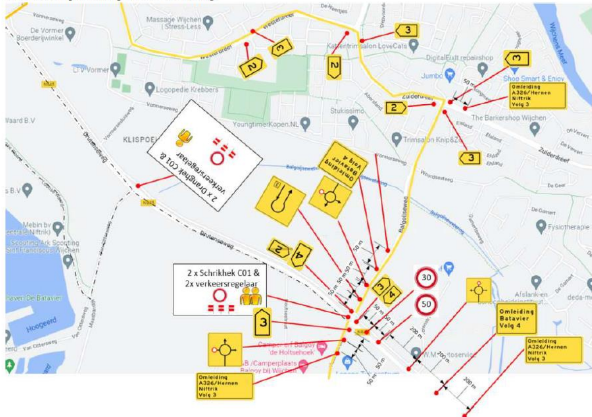
Detailtekening omleidingsroute N845 vervolg
