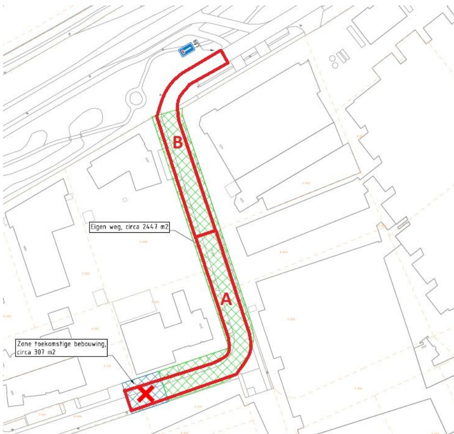
Figuur 2: Te onttrekken weggedeelte (A per direct, B per 1-2-2025)
