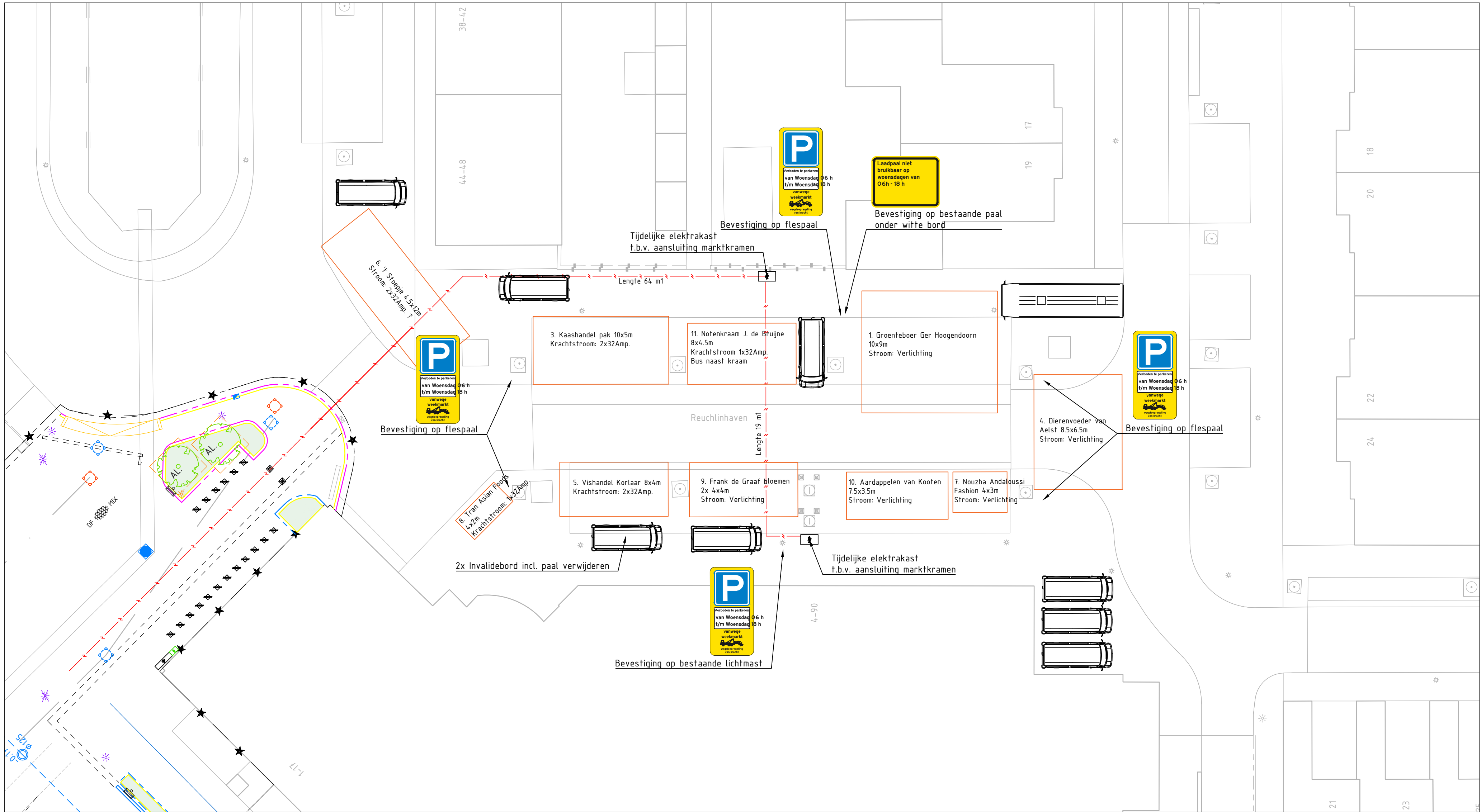
Tijdelijke situatie marktkramen Reuchlinhaven SCHAAL 1 : 200
