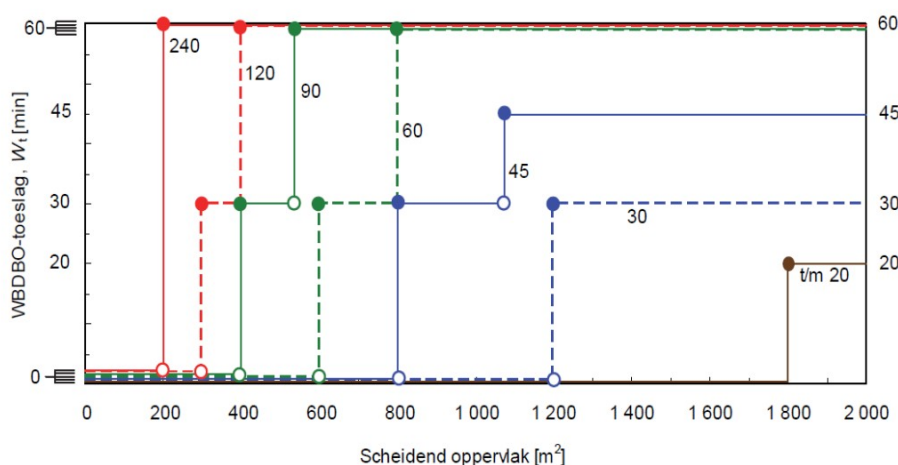
Figuur 3 Grafiek voor de WBDBO-toeslagbepaling volgens NEN 6060
