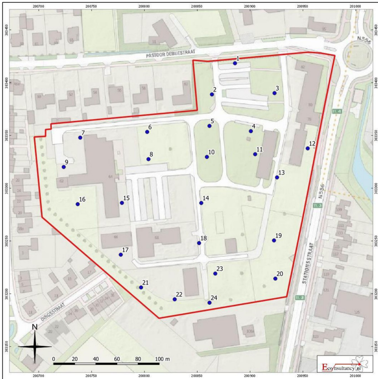
Figuur 17. Boorpuntenkaart 63
