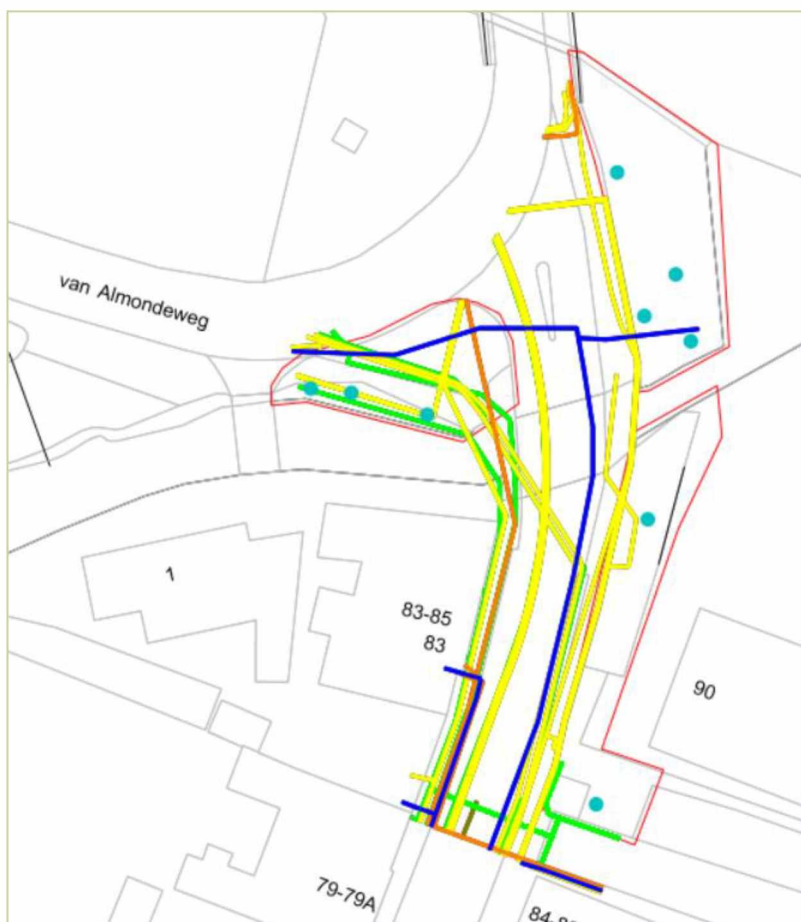
Locatie van de onderzoeksbomen inclusief aanwezige kabels en leidingen.
