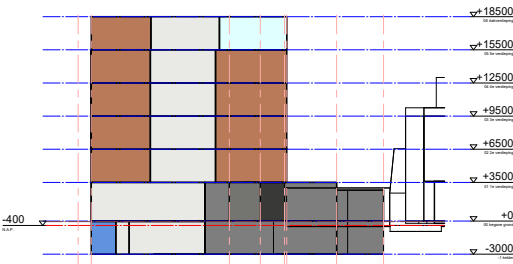
Doorsnede
