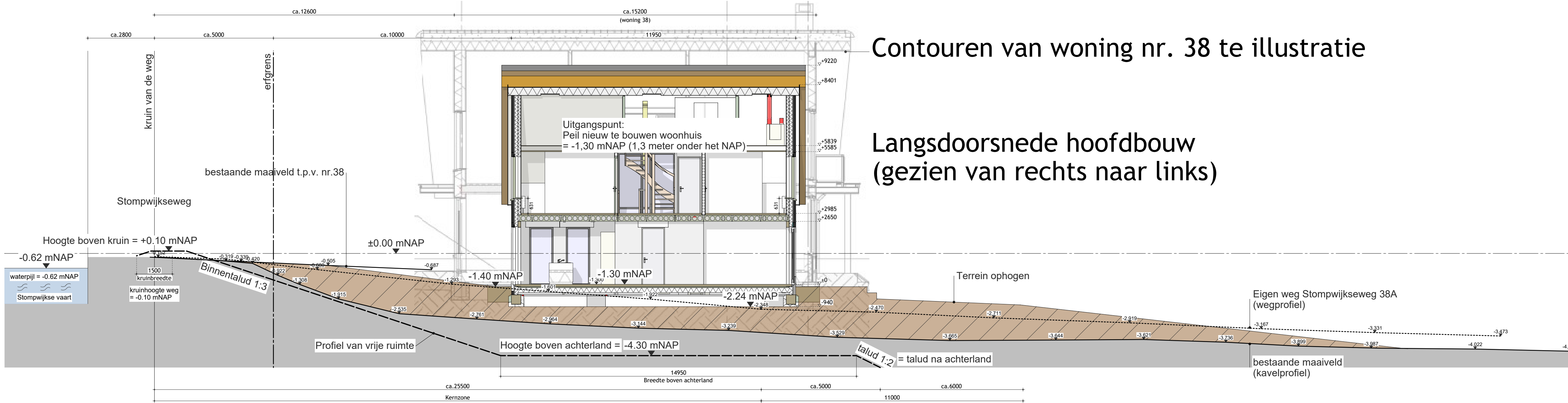
Dwarsprofiel t.o.v. profiel van vrije ruimte van de waterkering met maatvoering t.o.v. NAP Kern- en beschermingszone van de ter plaatse aanwezige regionale waterkering van de Nieuwe Driemanspolder (Hoogheemraadschap van Rijnland)
