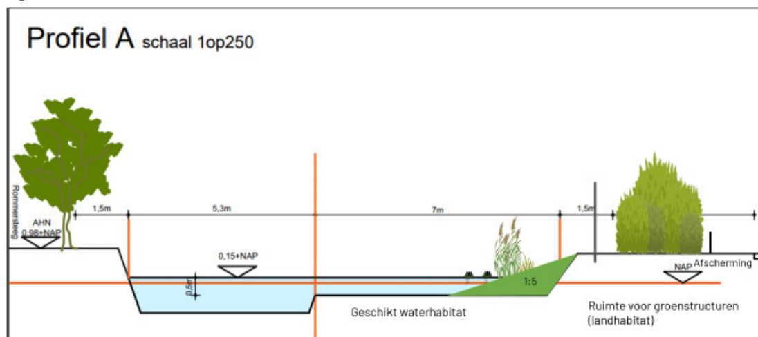
Figuur . Schematische weergave van profiel A (na de graafwerkzaamheden) inclusie natuurvriendelijke oever.
