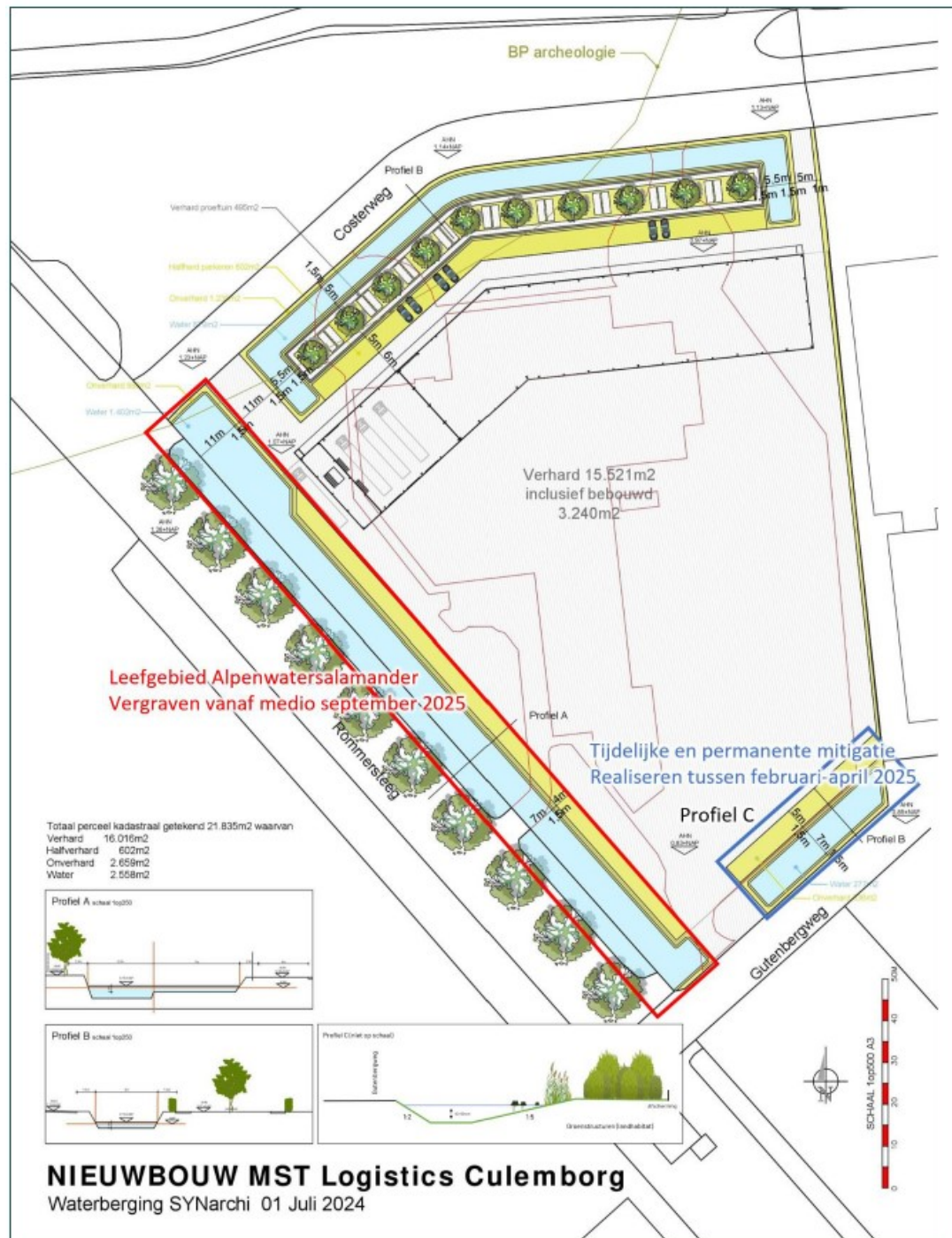
Figuur 3. Weergave van de toekomstige situatie inclusief de fasering in de aanleg.
