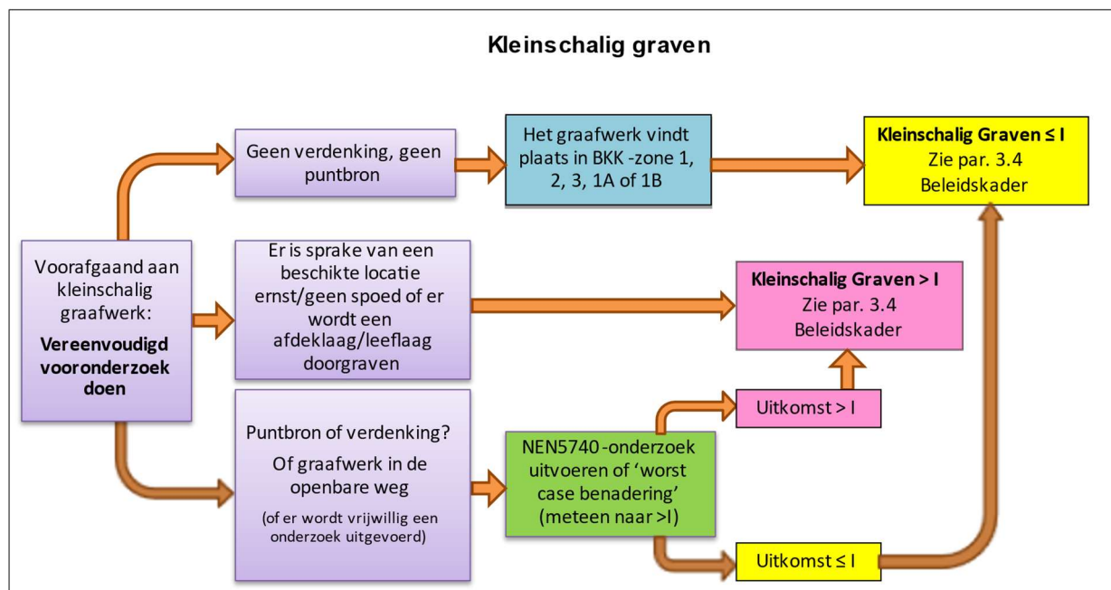
Figuur 3.2 Schematisch overzicht Kleinschalig graven
