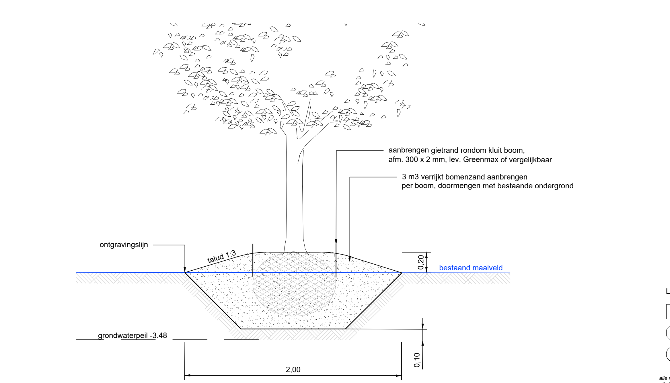
Normalprofil 3: grondwerk nieuwe heesters- en bomen schaal 1:20
