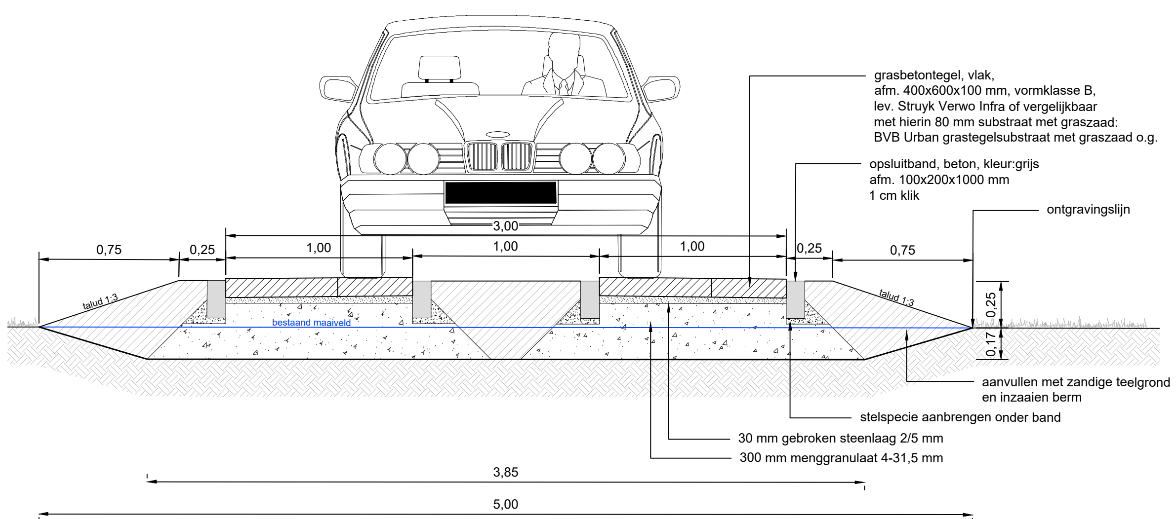
Normalprofil 2: nieuwe situatie karrespoor schaal 1:20
