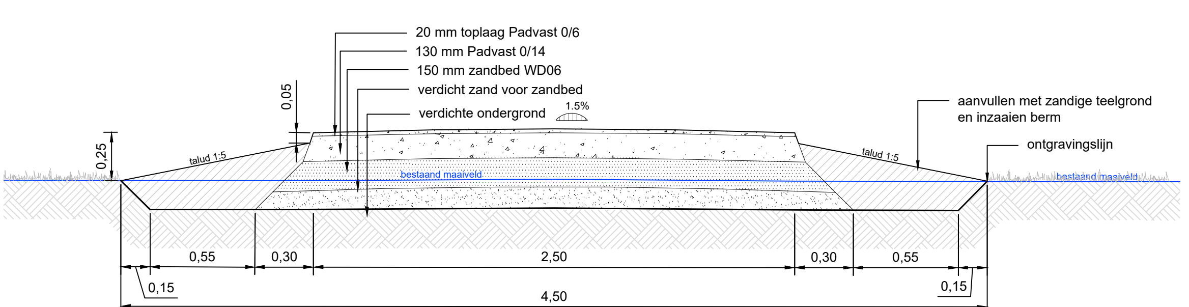
Normalprofil 1b: nieuwe situatie Padvast schaal 1:20
