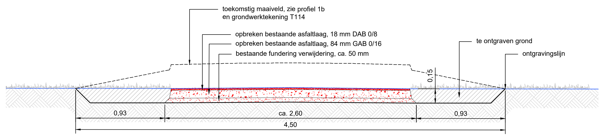
Normalprofil 1a: bestaande situatie Asfaltpad schaal 1:20
