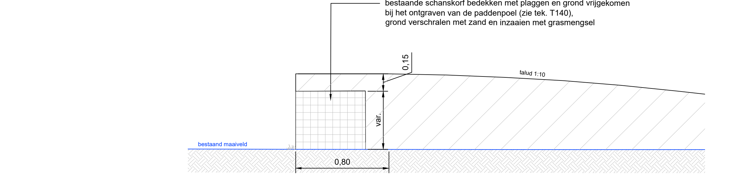
Normalprofil 4: nieuwe situatie heuvel schanskorf schaal 1:20
