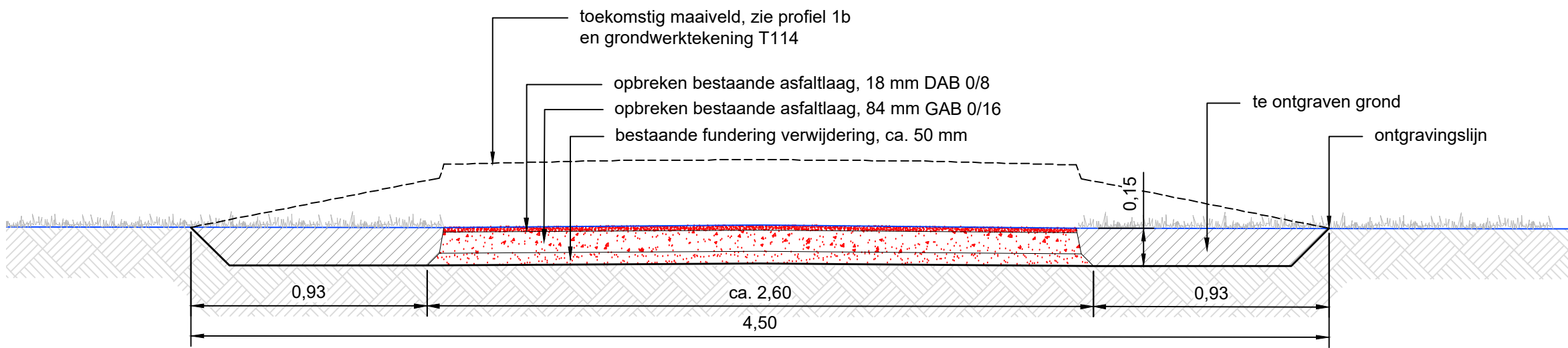
Normaalprofiel 1a: bestaande situatie asfaltpad schaal 1:20
