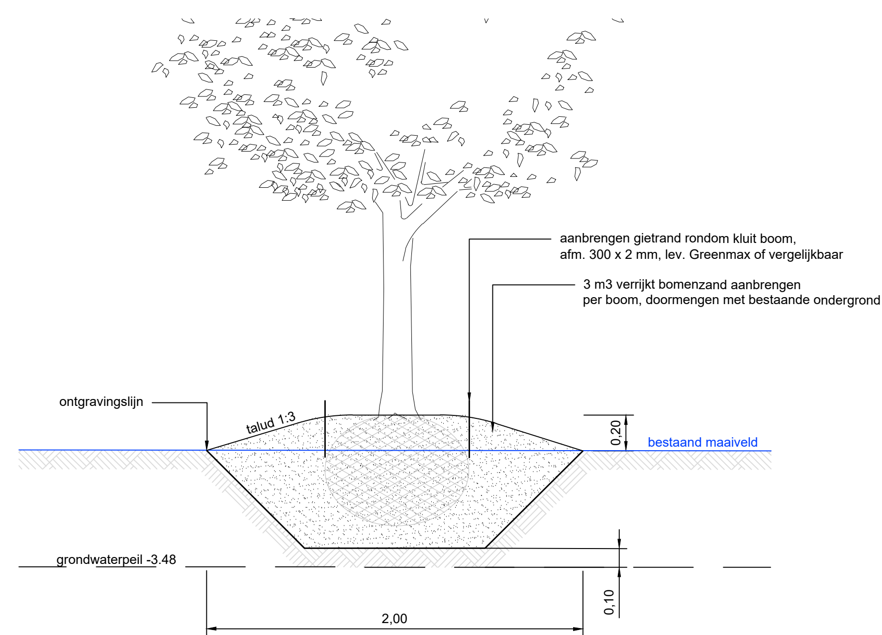
Normaalprofiel 3: grondwerk nieuwe heesters- en bomen schaal 1:20
