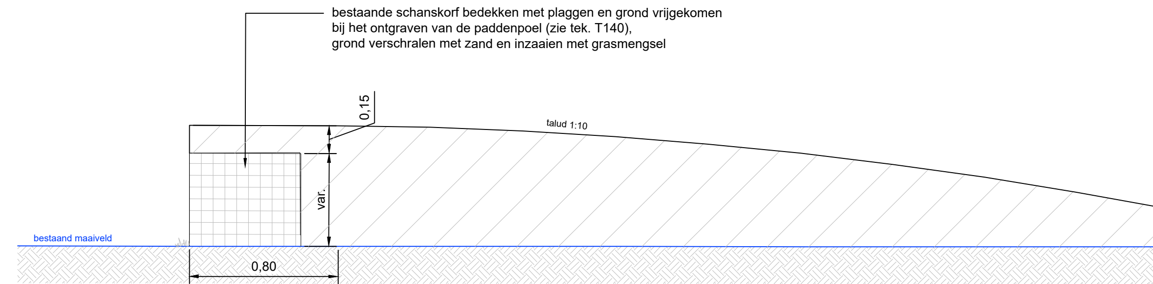
Normaalprofiel 4: nieuwe situatie heuvel schanskorf schaal 1:20
