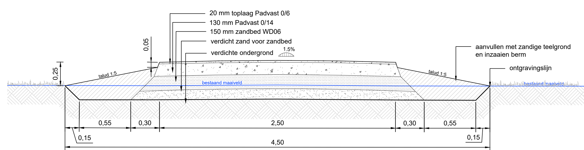
Normaalprofiel 1b: nieuwe situatie padvast schaal 1:20
