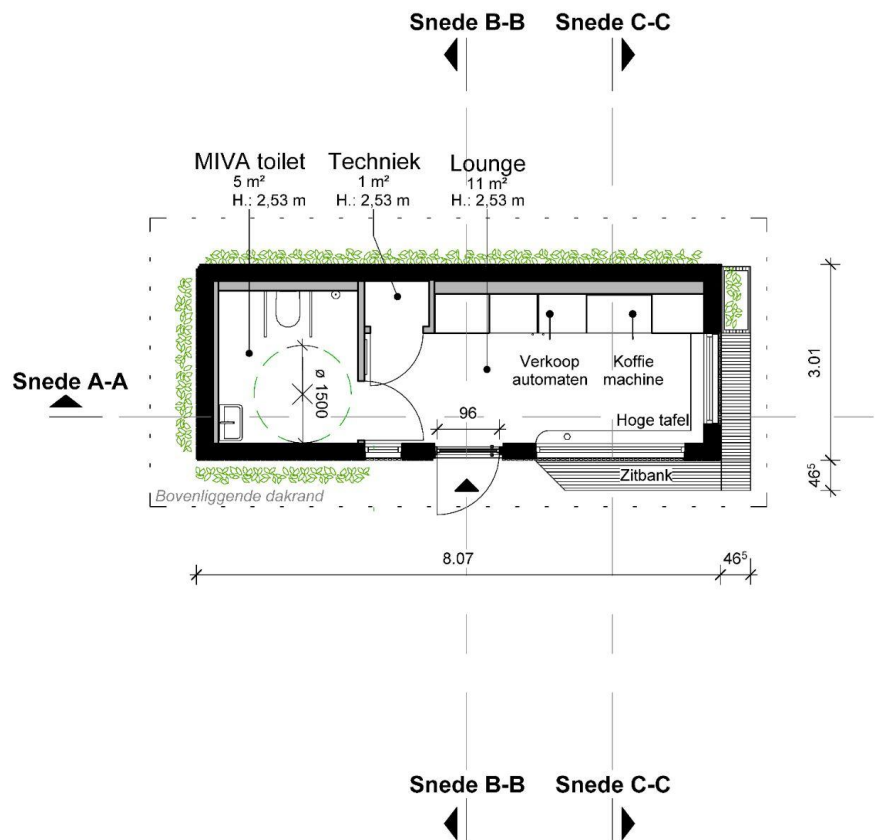
Grondplan
