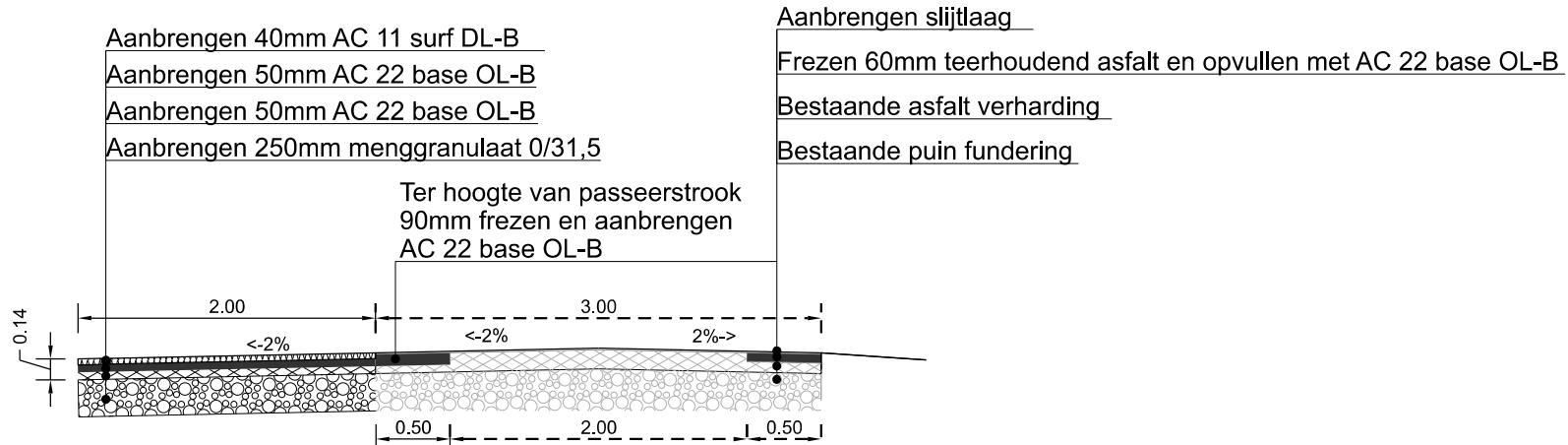
Oostelijk deel principe profiel Schaal 1:50
