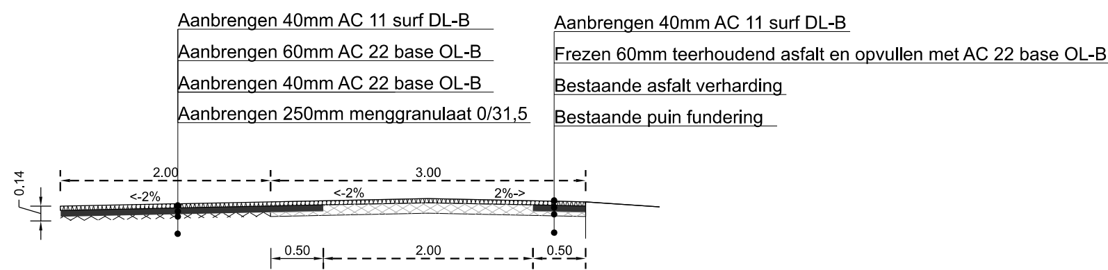
Westelijk deel principe profiel Schaal 1:50
