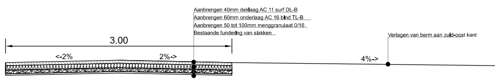
Principe profiel Schaal 1 : 50
