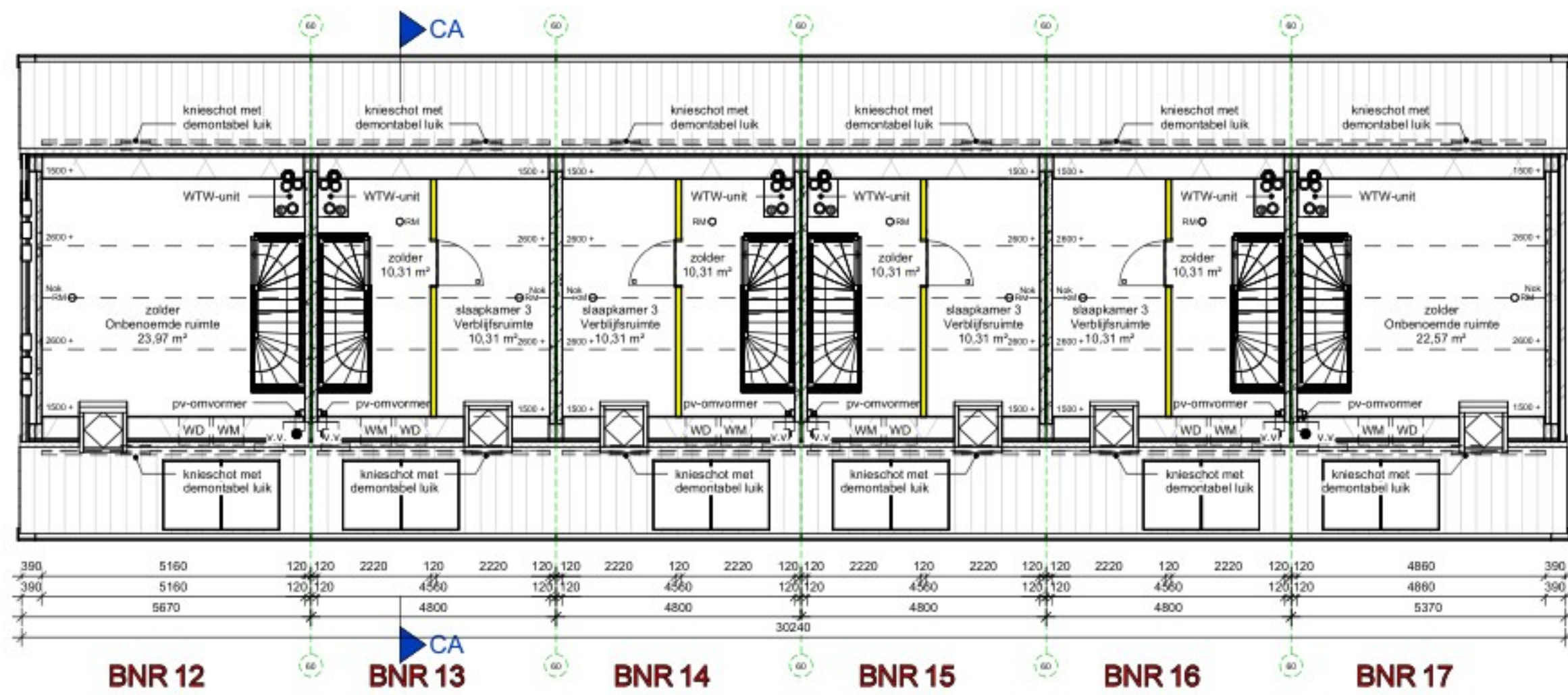
2e verdieping
