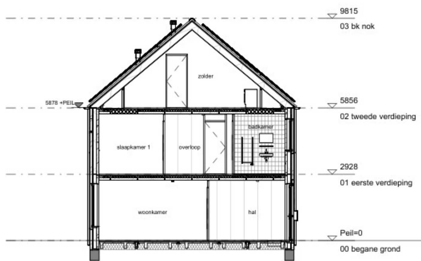
doorsnede CA
