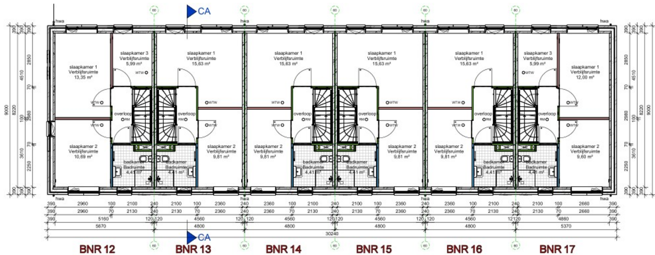
1e verdieping
