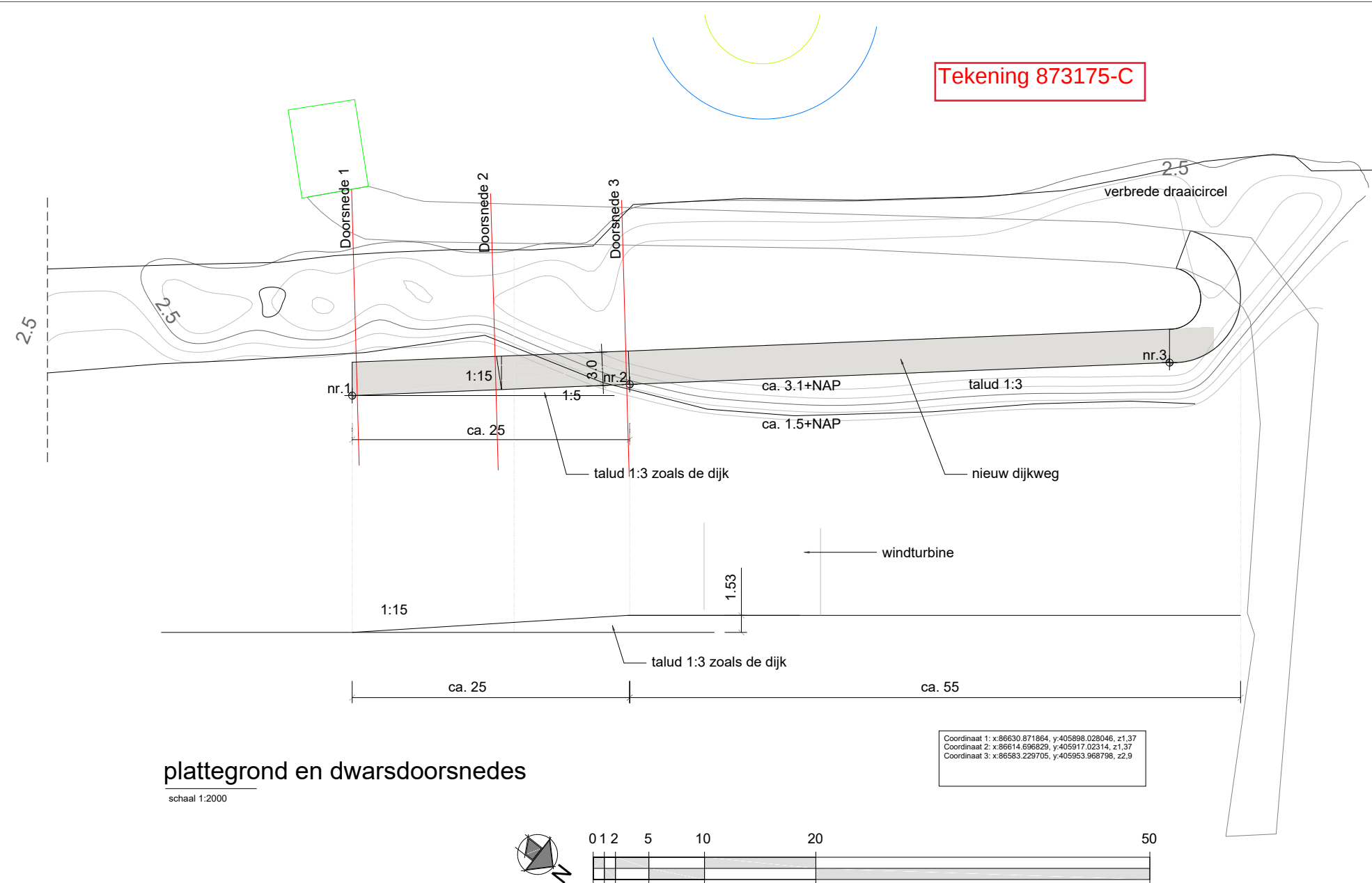
Doorsnede 1
