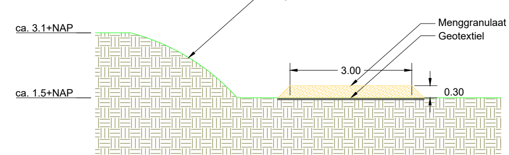
Doorsnede 1
