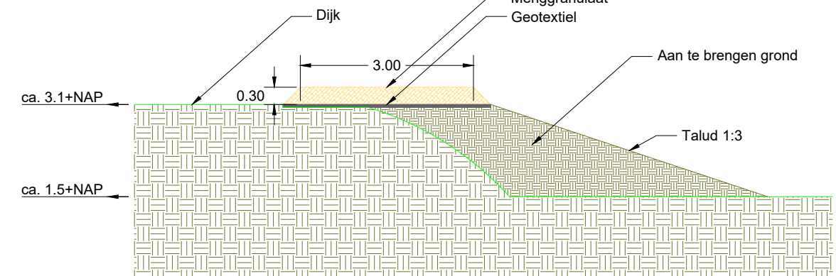
Doorsnede 3
