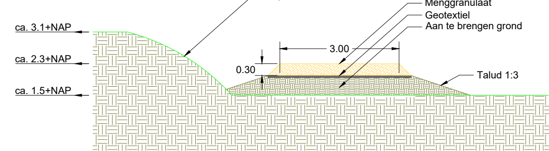
Doorsnede 2
