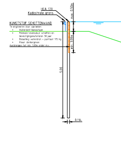
Detail 4B: Doorsnede Principeprofiel keerwand HEA120 Schaal 1:5
