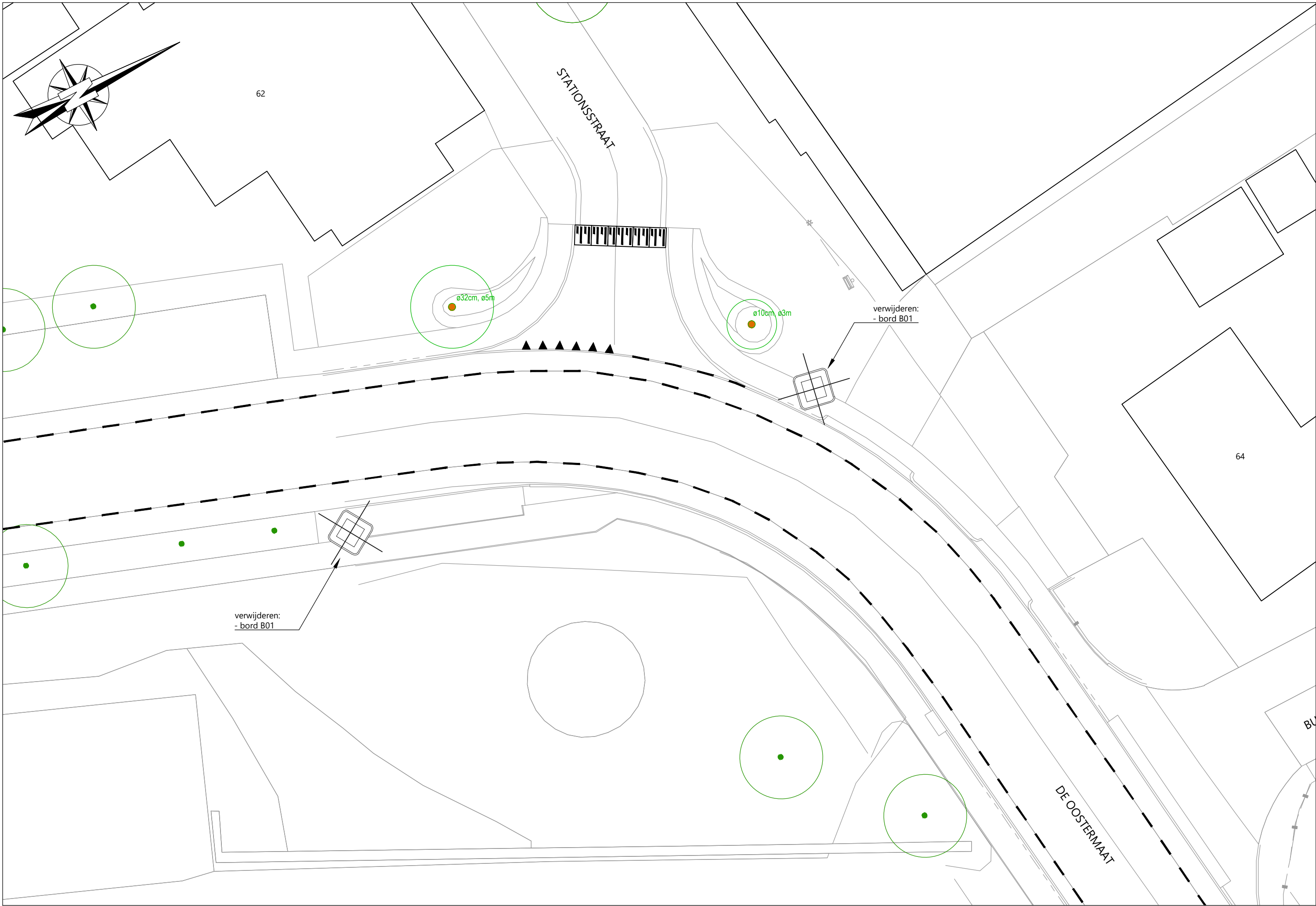
DETAIL C - DE OOSTERMAAT - STATIONSSTRAAT
