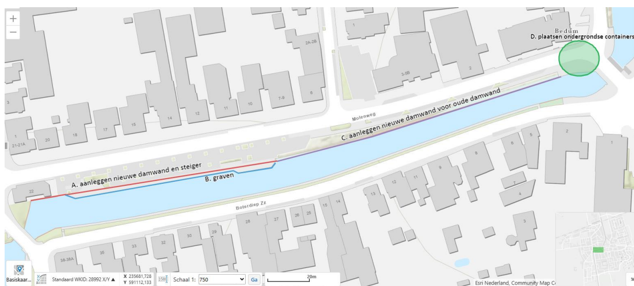
Figuur 1: De rode lijn geeft globaal de locatie weer van de nieuwe damwand en daaraan gelegen steiger (A), het oppervlak tussen de rode en blauwe lijn wordt gegraven (A en B), de paarse lijn geeft globaal de locatie weer van een nieuwe damwand die voor de oude damwand wordt geplaatst (C) en binnen de groene cirkel worden ondergrondse containers geplaatst (D).
